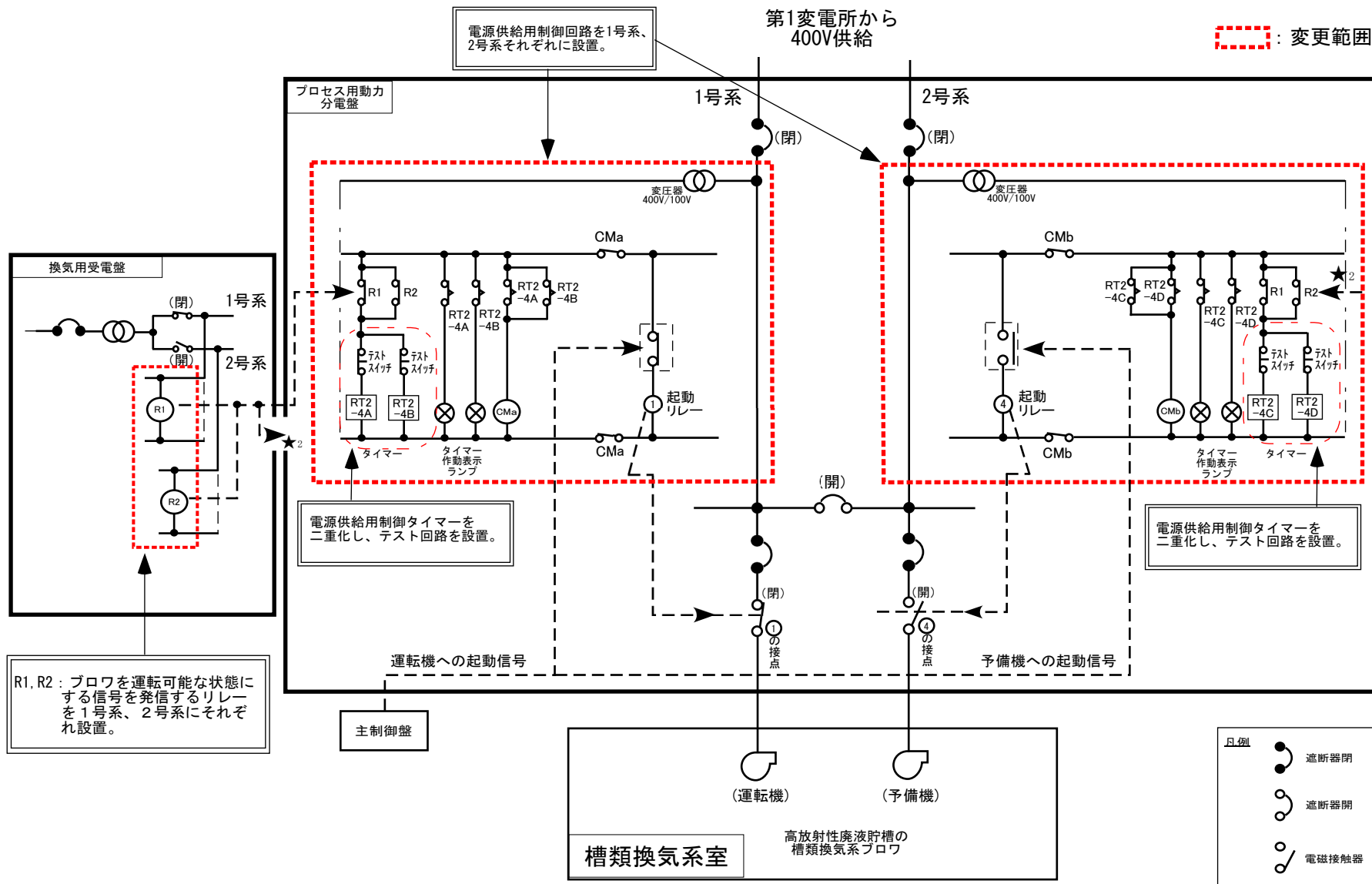
図-3. 変更後の槽類換気系ブロウ起動系統概要図
