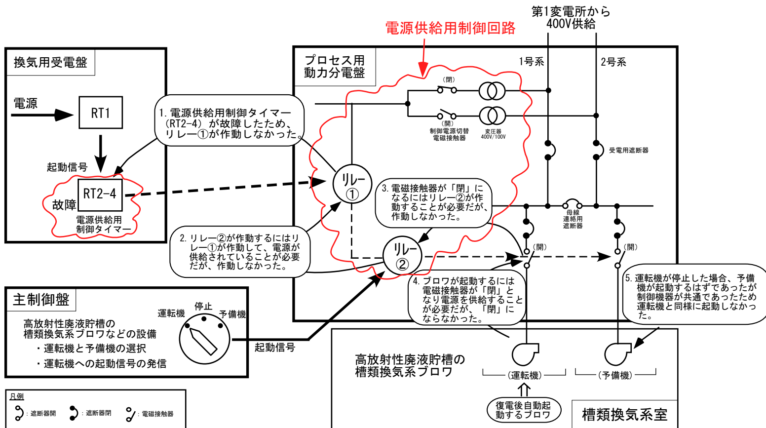
図-1. 分離精製工場 槽類換気系概略図 (事象対象機器)
