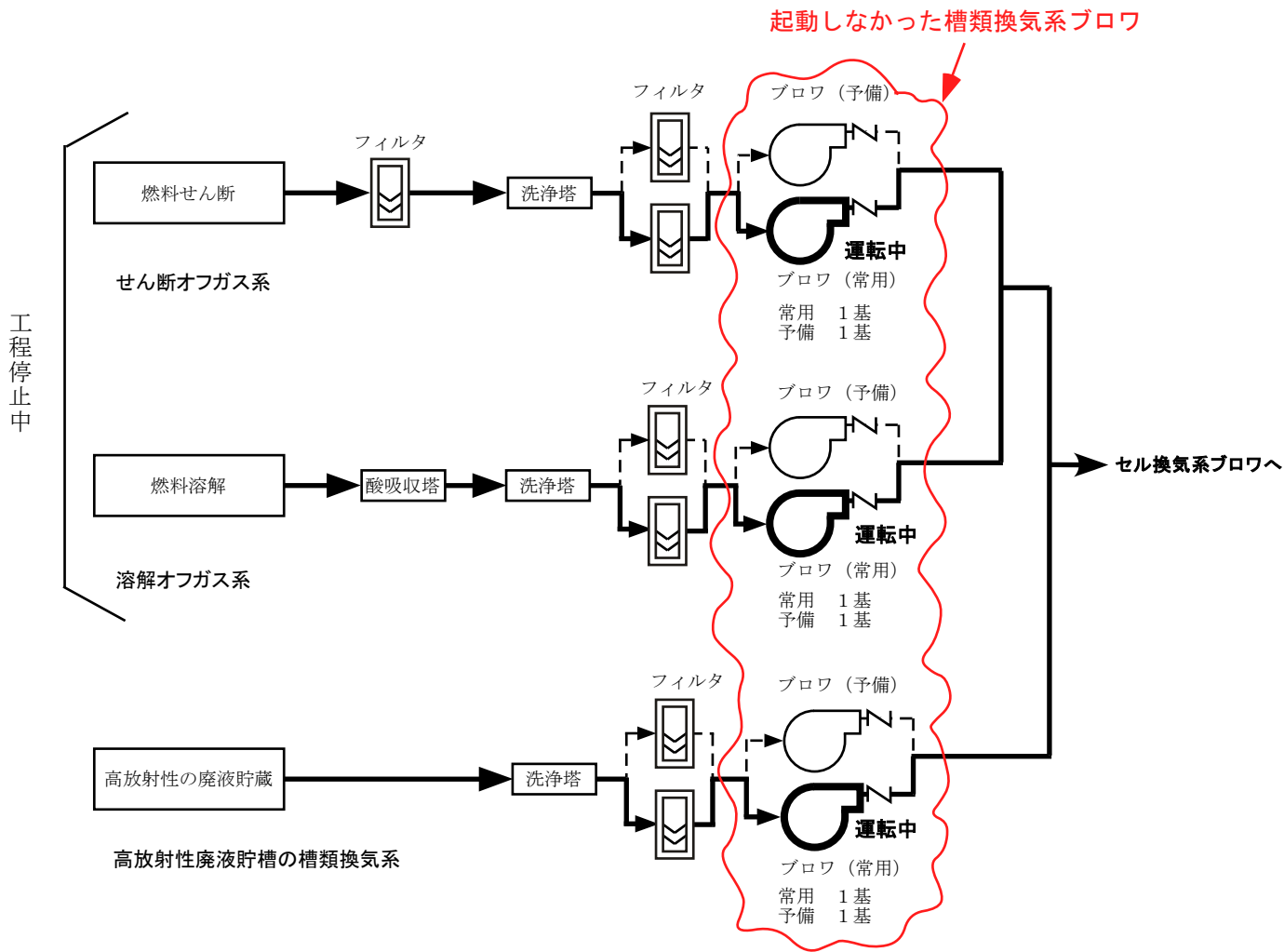
図-1. 分離精製工場 槽類換気系概略図 (事象対象機器)
