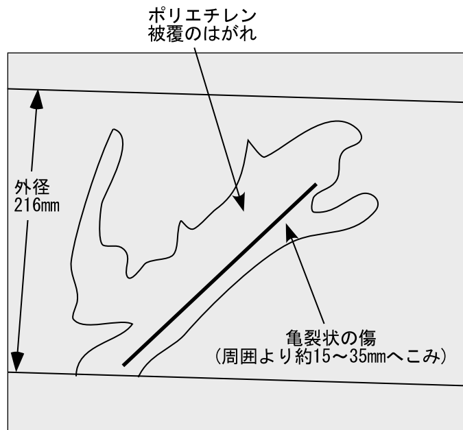
北側面から見た漏えい箇所の模式図
