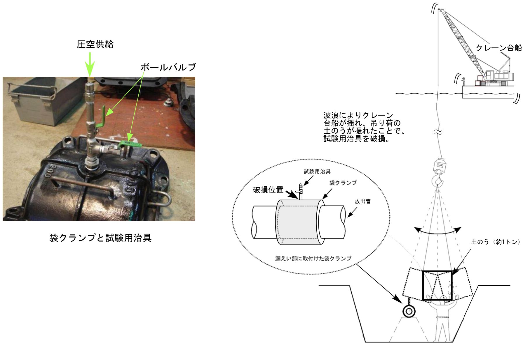
図-1 土のうによる袋クランプの試験用治具の破損の概要図
