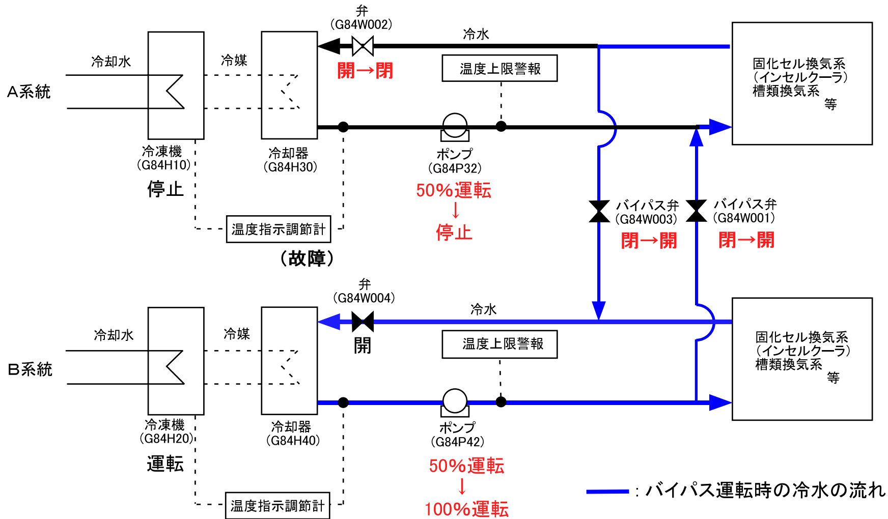
図-2 冷水設備運転状態(バイパス運転時)
