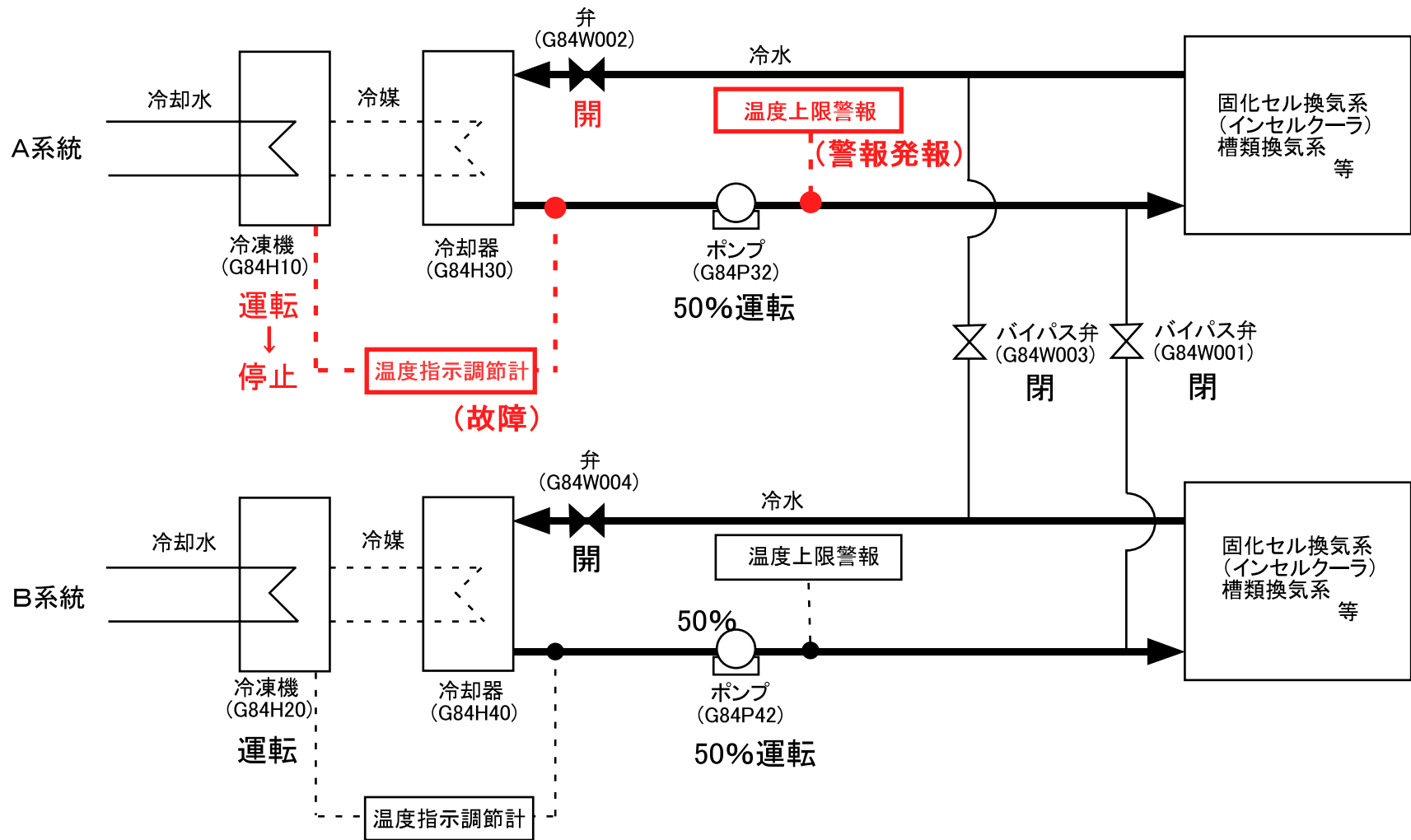
図-1 冷水設備運転状態(事象発生時)
