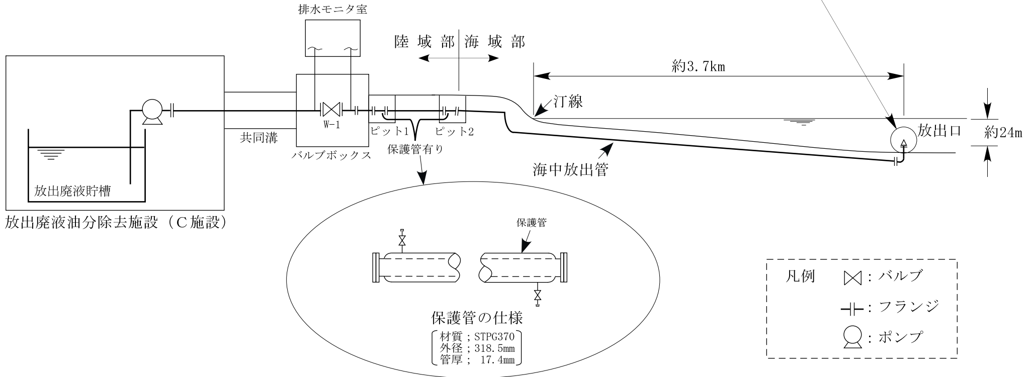
図 - 1 海中放出設備概要図
