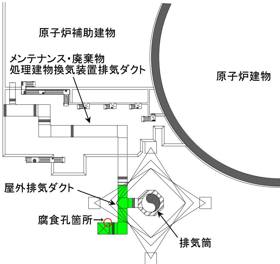
原子炉補助建物(屋上)平面図
