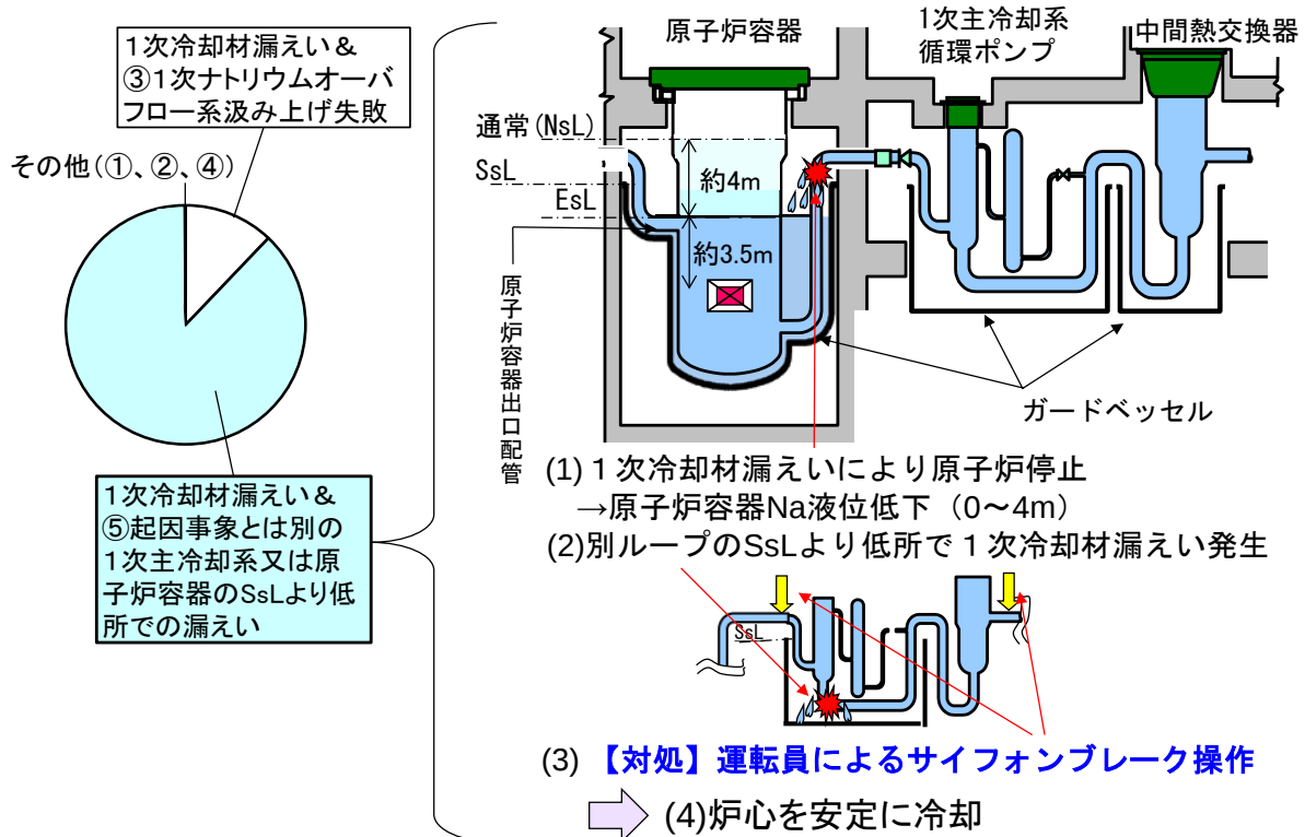
図 4.2.1-4 原子炉容器液位確保機能喪失の事故シーケンス抽出
