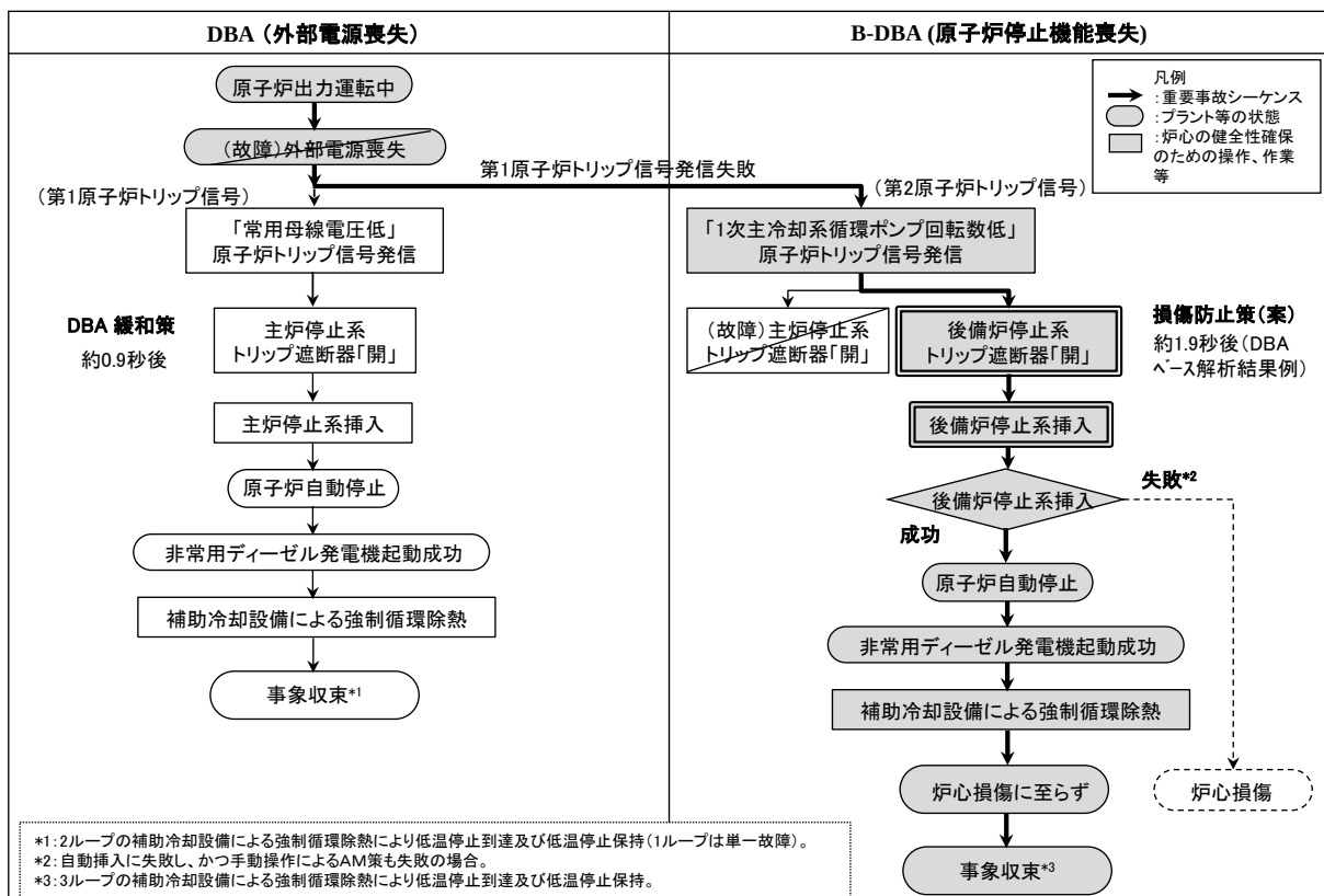
付録 5.1 図-11 原子炉停止機能喪失の重要事故シーケンス
