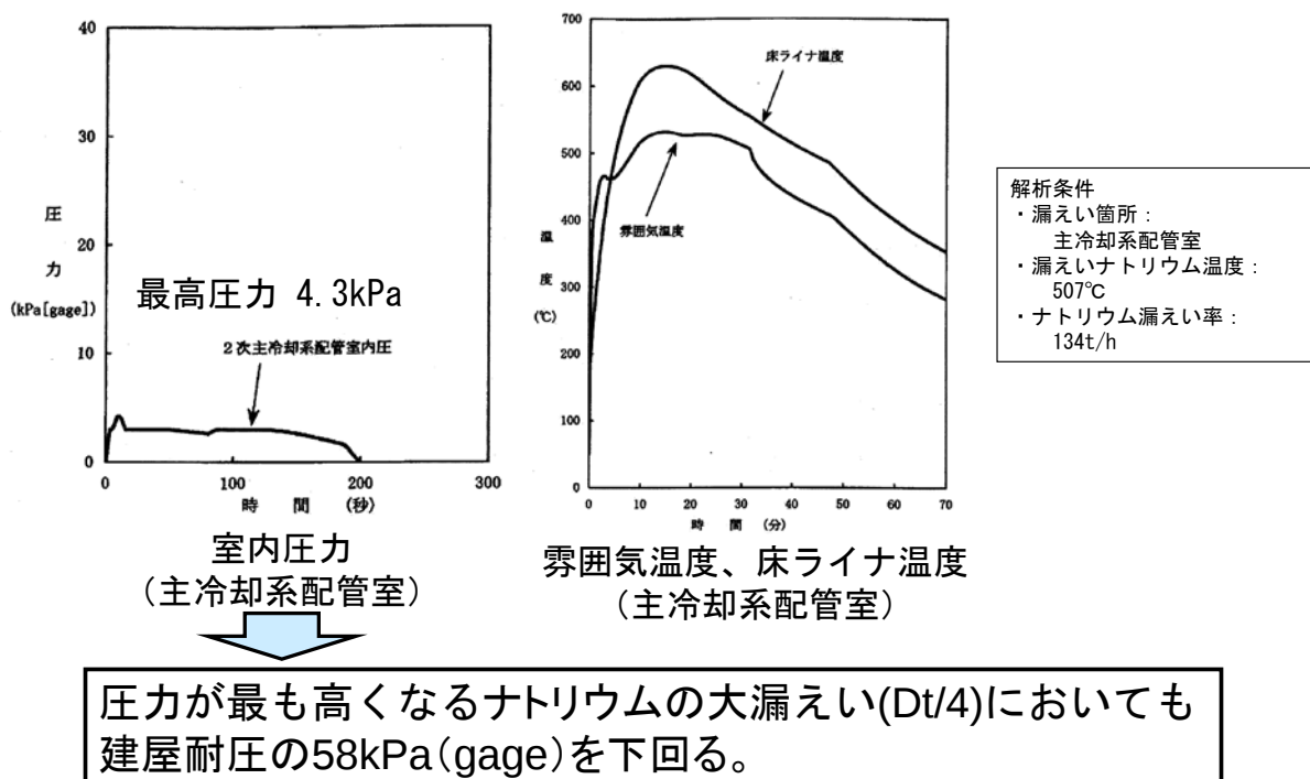
付録 4.2 図-5 設計基準での評価結果(ナトリウムの流出・床ライナ上の移送過程の熱的影響)
