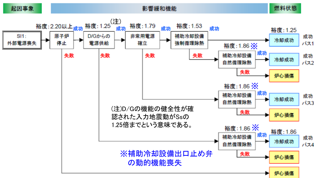
付録 5.1 図-7 耐震裕度に対するイベントツリー
