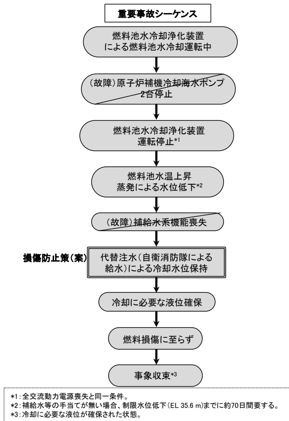
付録 5.1.2 図-7 燃料池の重要事故シーケンス
