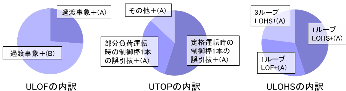
図 4.2.4-1 ATWS の事故シーケンスの内訳と選定された重要事故シーケンス
