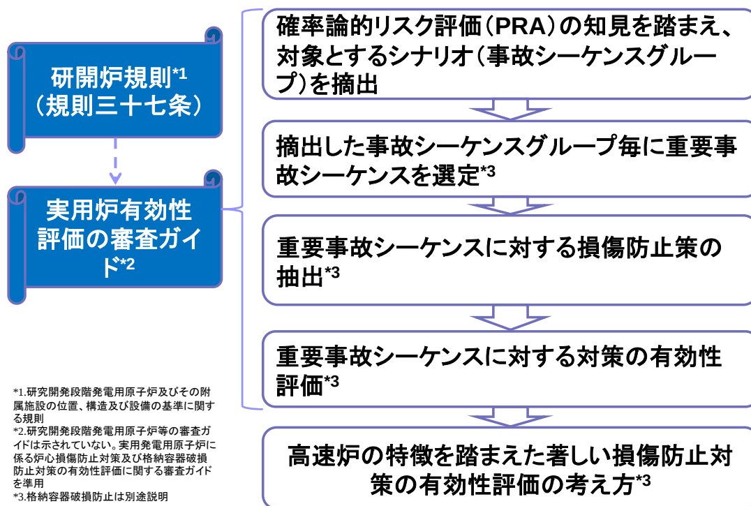
付録 5.1 図-1 損傷防止策の有効性評価の手法
