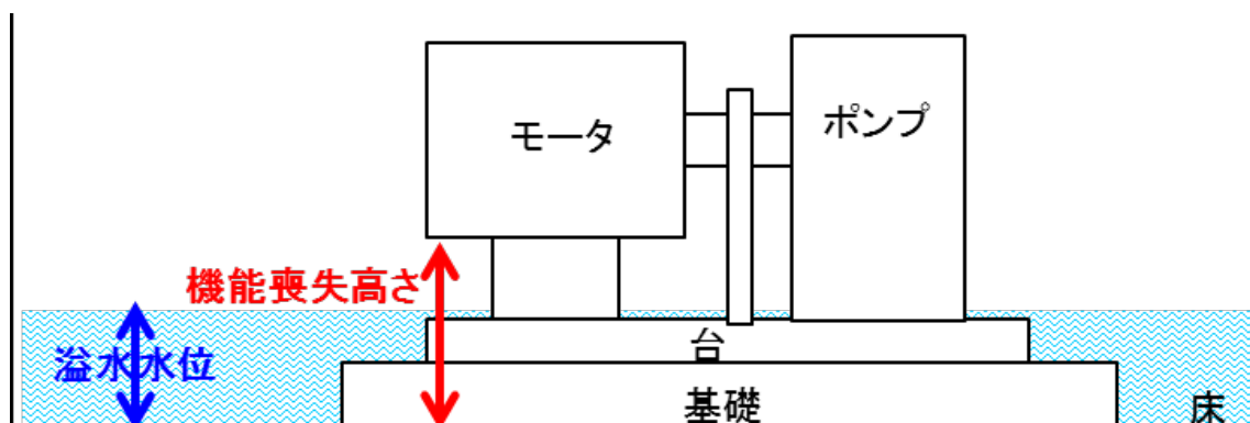
図 3.6-1 没水評価イメージ
