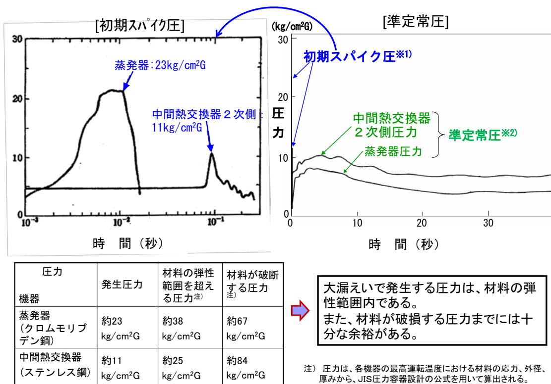
付録 4.1 図-9 設計基準として想定する漏えい規模での発生圧力及び影響評価
