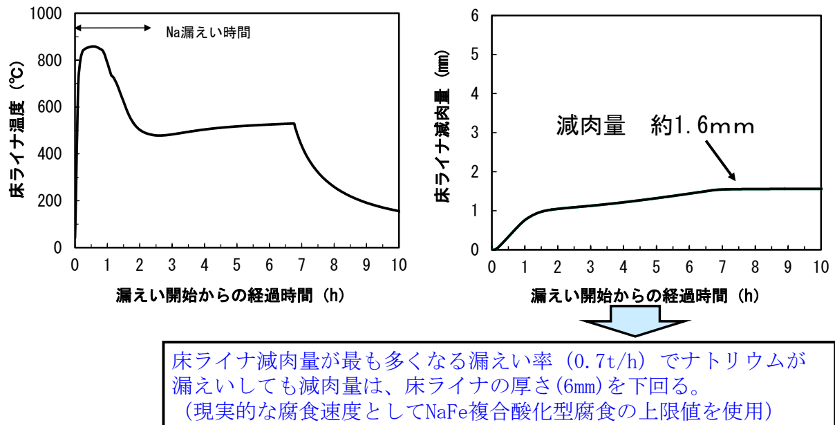
付録 4.2 図-12 全交流電源喪失状態での評価結果（床ライナ減肉量）
