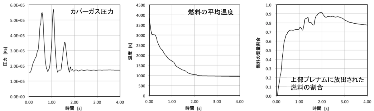
付録 5.2 図-16 「もんじゅ」炉心膨張挙動の解析結果
