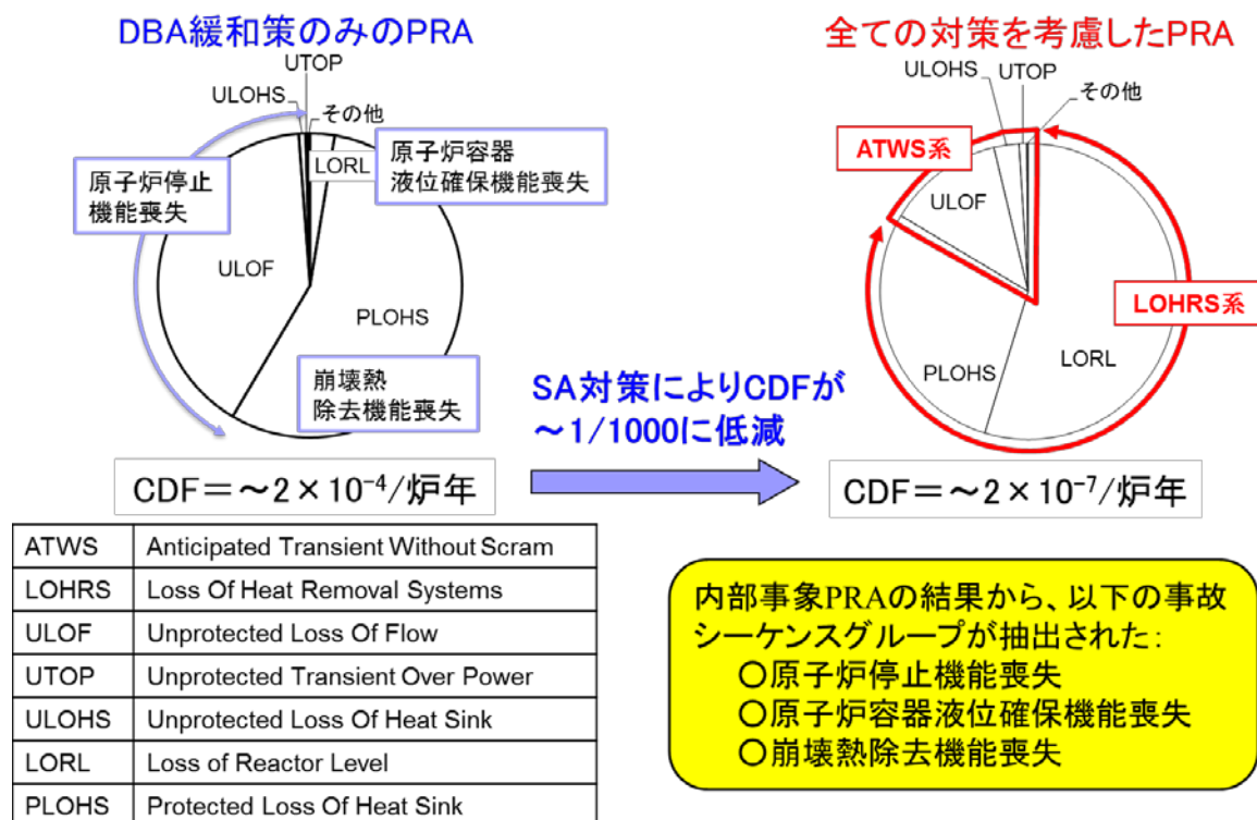
図 4.2.1-1 内部事象から選定される事故シーケンスグループ(レベル1PRAの結果)
