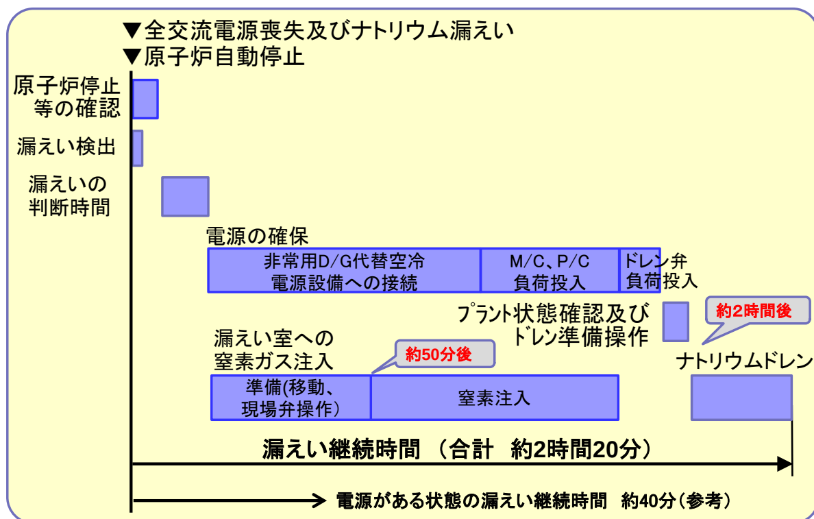
付録 4.2 図-10 全交流電源喪失状態でのナトリウム漏えい対応手順
