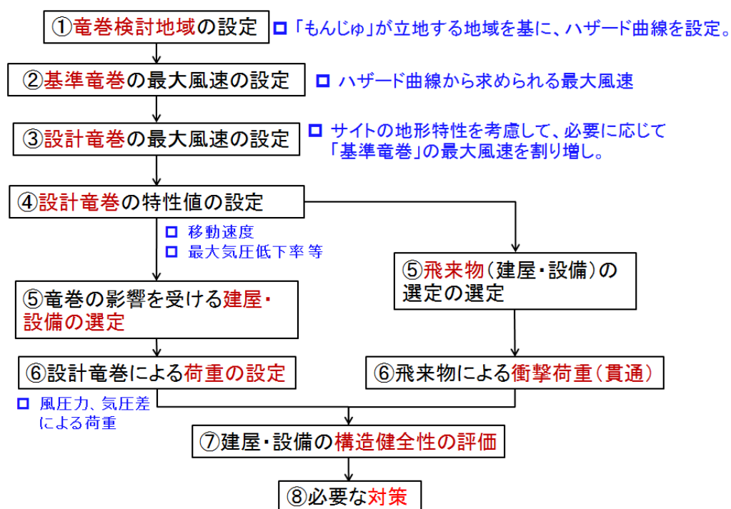
図 5.1-2 竜巻の評価手順
