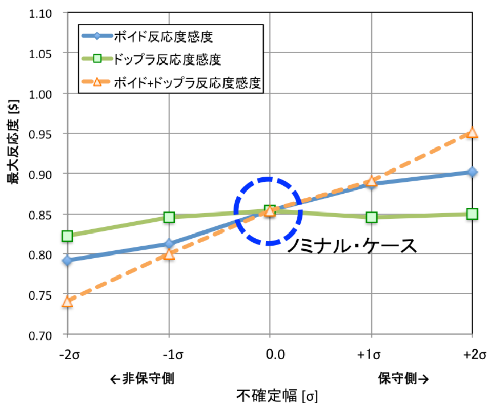
付録 5.2 図-5 「もんじゅ」起因過程における反応度係数不確かさの影響
