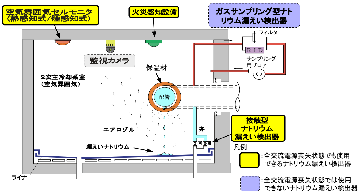
付録 4.2 図-9 全交流電源喪失状態でのナトリウム漏えい検出
