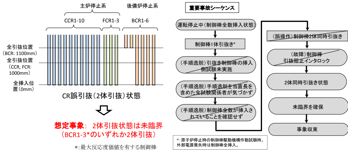
図 4.2.3-2 運転停止中の制御棒挿入状態
