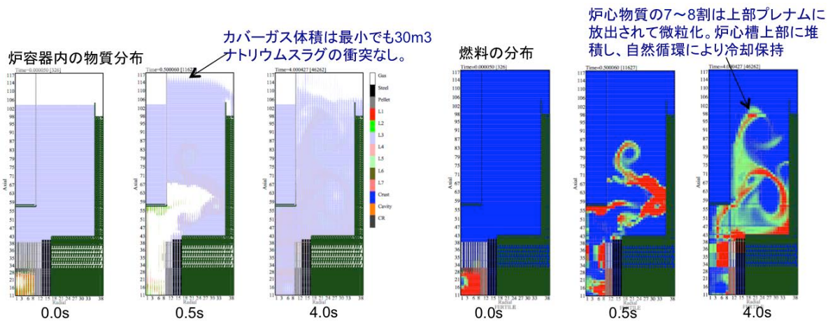
付録 5.2 図-15 「もんじゅ」炉心膨張挙動における上部プレナム内の物質分布
