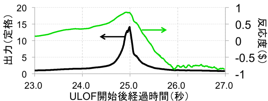
付録 5.2 図-4 「もんじゅ」起因過程ノミナルケースにおける出力と反応度の過渡挙動
