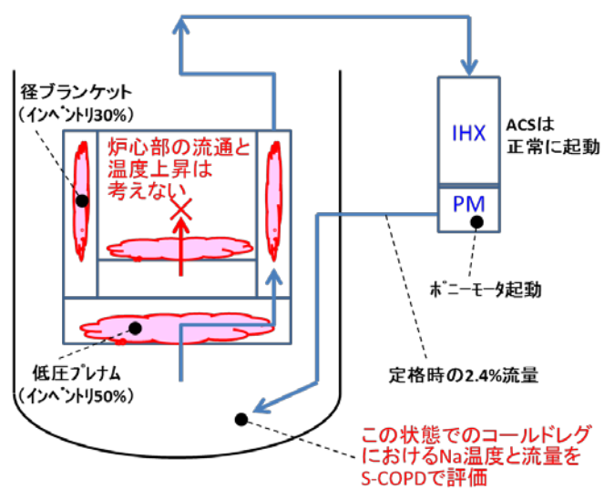
付録 5.2 図-17 「もんじゅ」冷却過程における冷却材流量評価体系
