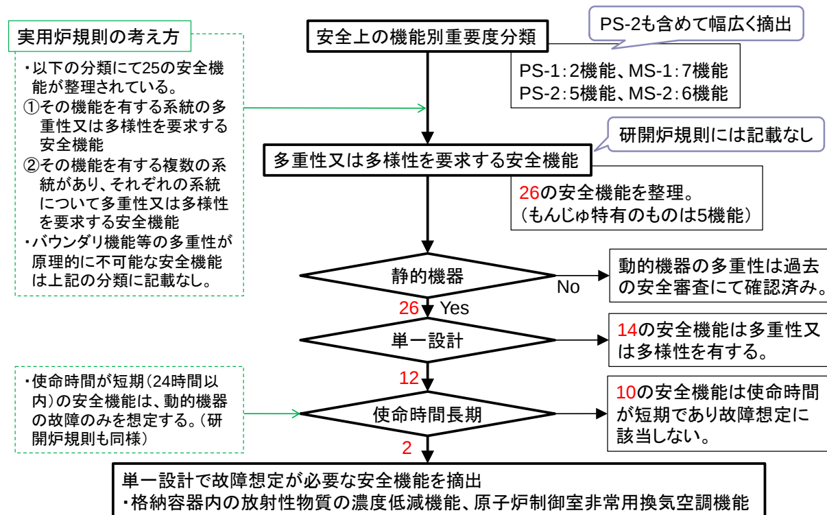
付録3 図-1 単一設計で故障想定が必要な安全機能の抽出に関する検討フロー
