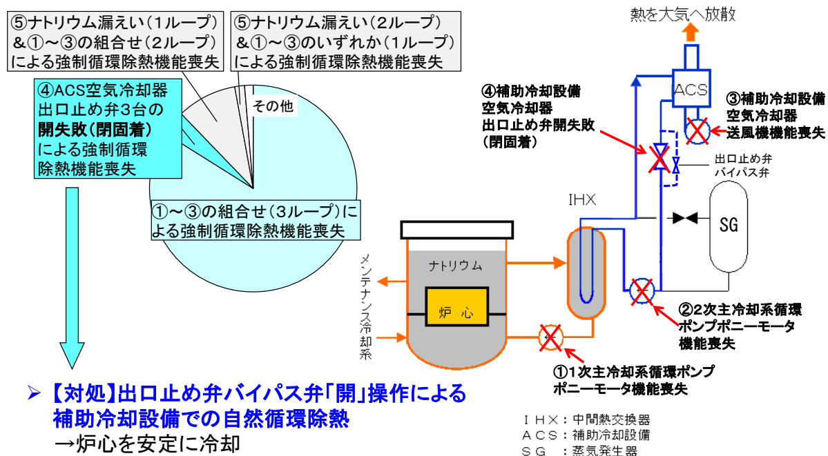
付録 5.1 図-6 崩壊熱除去機能喪失の事故シーケンス抽出
