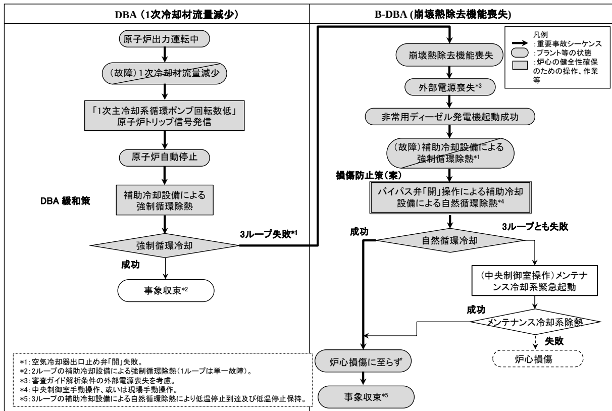
付録 5.1 図-13 崩壊熱除去機能喪失の重要事故シーケンス
