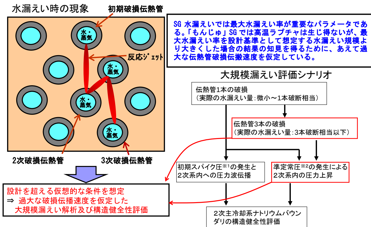
付録 4.1 図-10 設計基準の水漏えい規模を超える想定での評価の考え方
