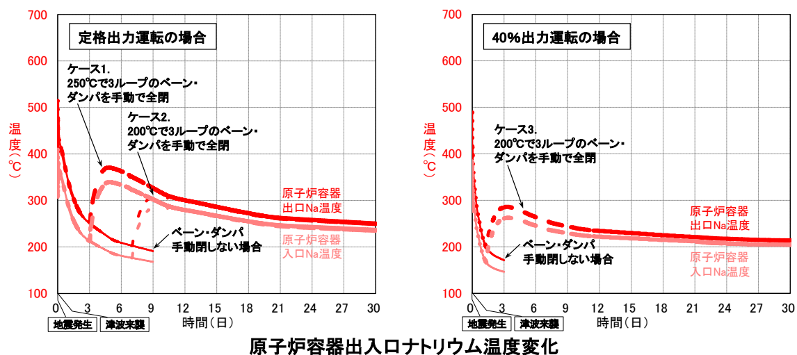
付録 5.1 図-18 全交流動力電源喪失時のプラント過渡応答解析結果例 (3/3)
