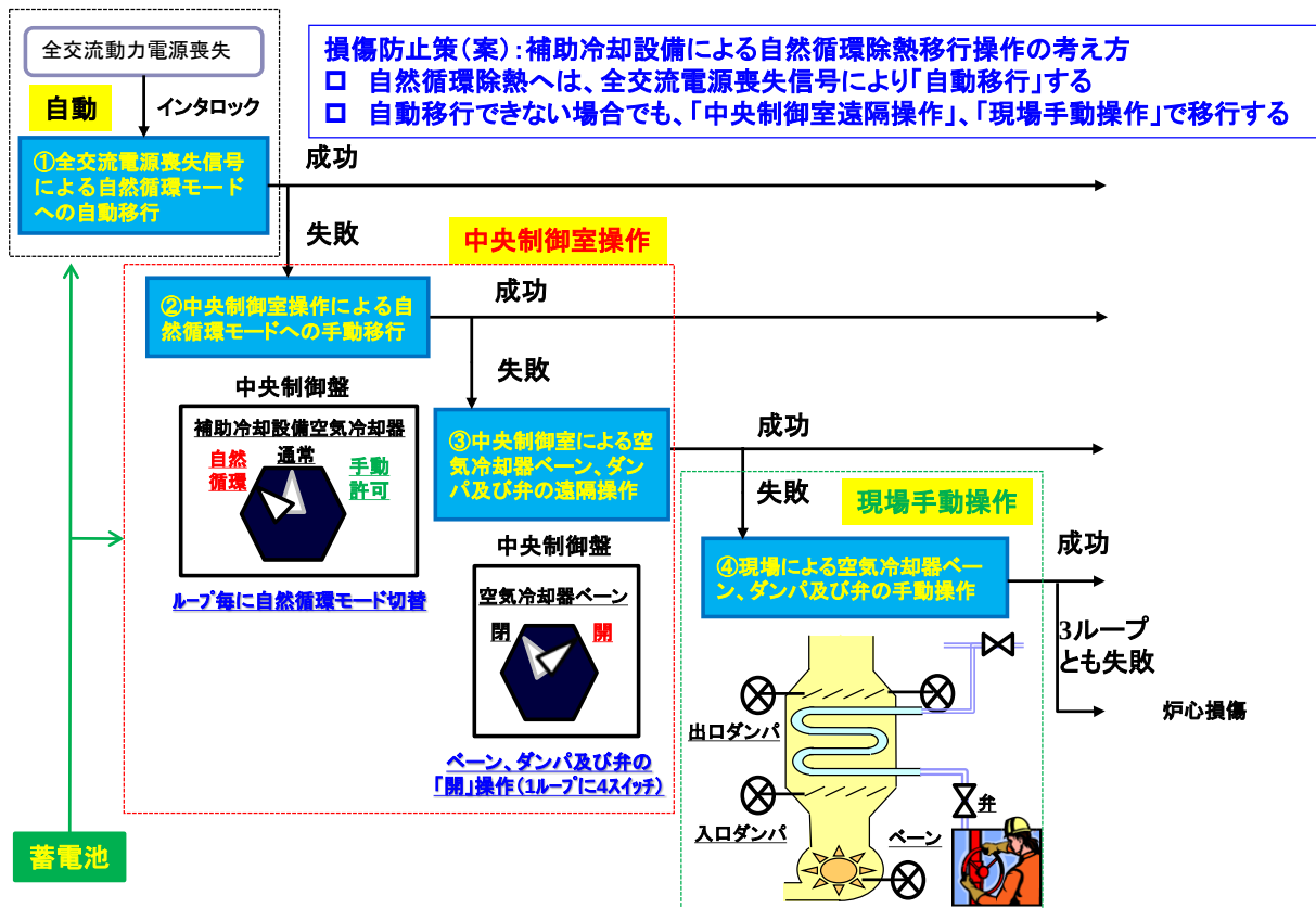
付録 5.1 図-15 補助冷却系の自然循環除熱移行操作
