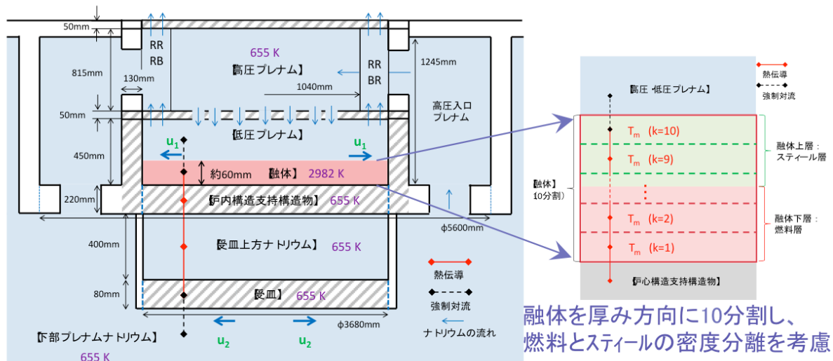
付録 5.2 図-19 低圧プレナムにおける炉心物質冷却保持挙動評価体系
