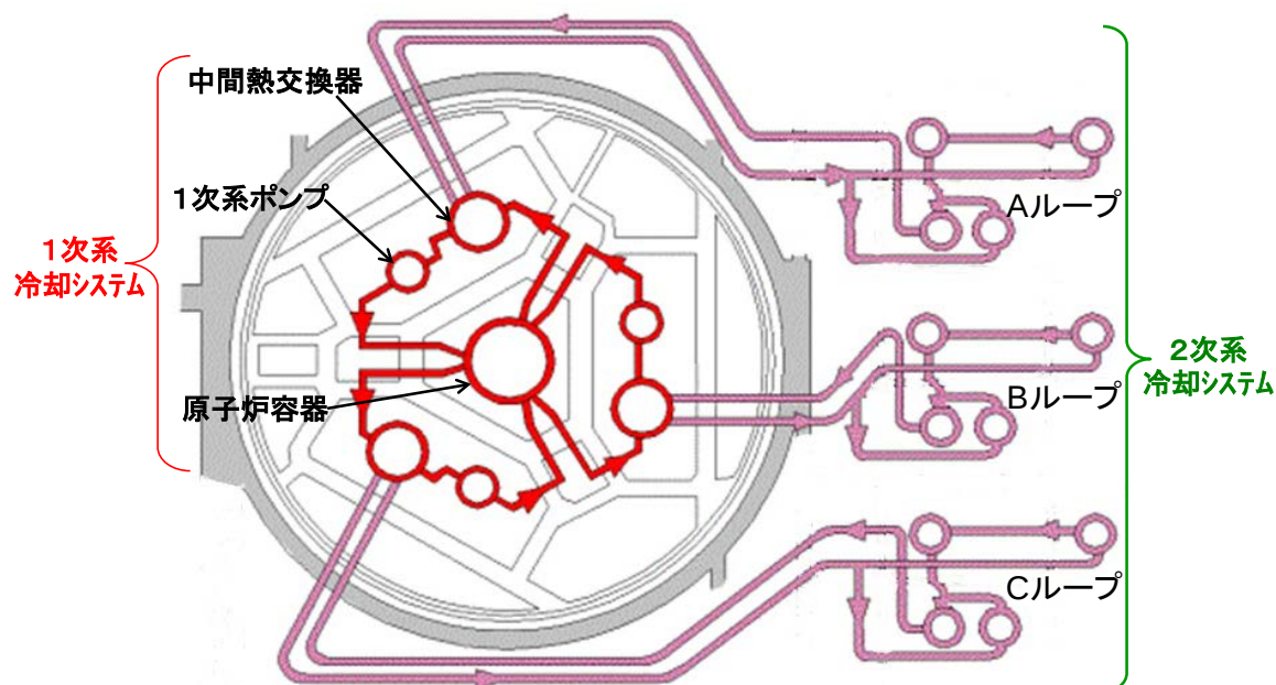
図 3.9-2 冷却系ループ構成(上面図)
