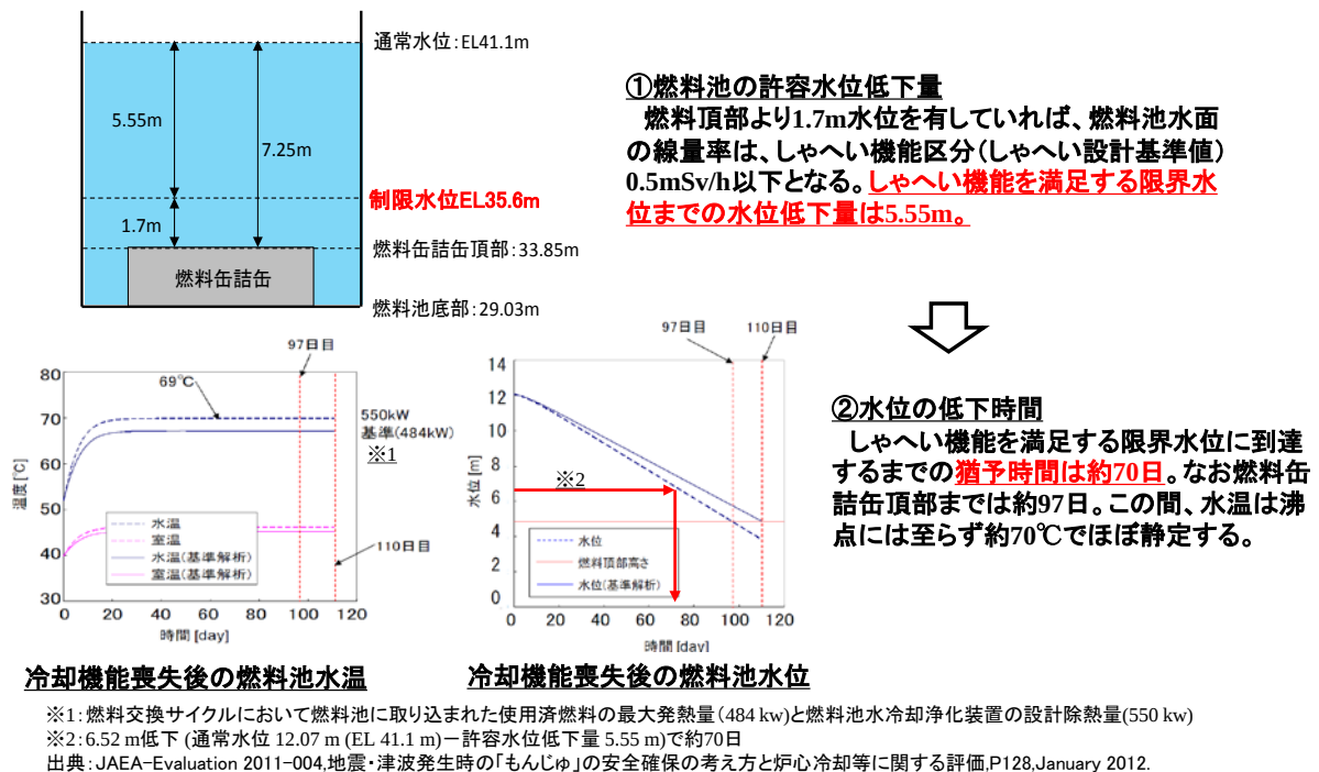
付録 5.1.2 図-8 燃料池水の水温及び水位の評価結果例
