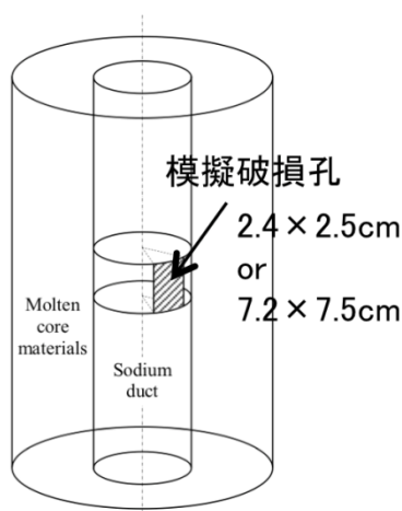
付録 5.2 図-11 「もんじゅ」CRGT 破損時の FCI 挙動解析体系
