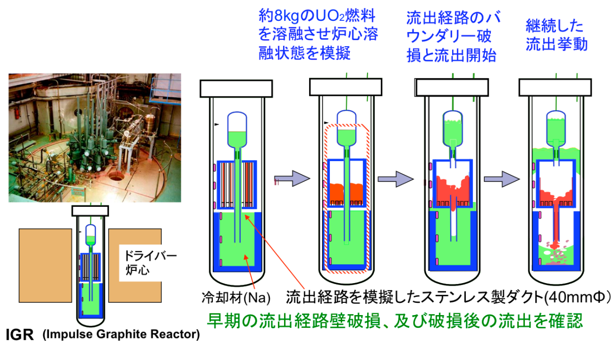
付録 5.2 図-7 EAGLE 試験の炉内試験例(ID-1 試験)
