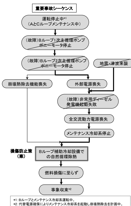
付録 5.1.3 図-4 運転停止中崩壊熱除去機能喪失(全交流動力電源喪失)の重要事故シーケンス
