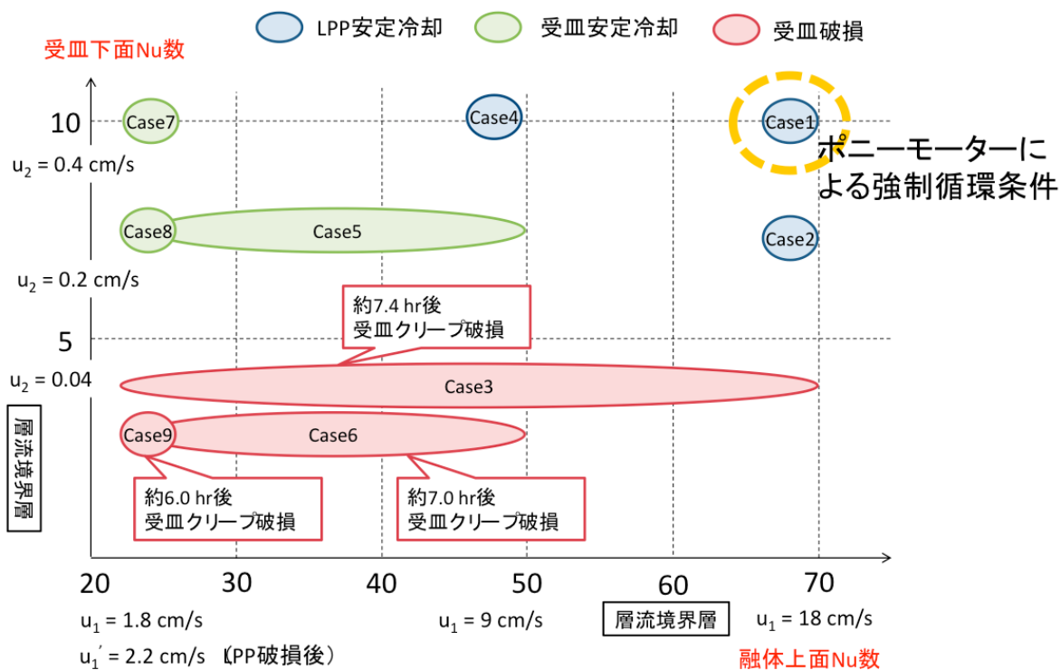
付録 5.2 図-20 低圧プレナムにおける炉心物質冷却保持挙動評価結果
