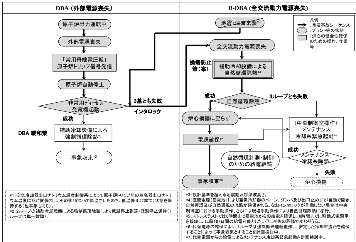
付録 5.1 図-14 全交流動力電源喪失の重要事故シーケンス
