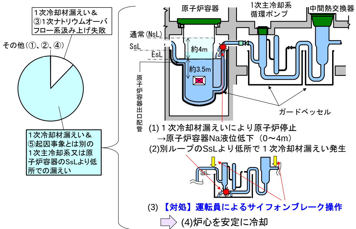
付録 5.1 図-5 原子炉容器液位確保機能喪失の事故シーケンス抽出
