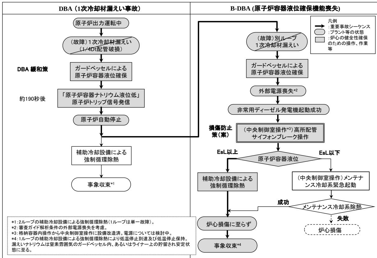
付録 5.1 図-12 原子炉容器液位確保機能喪失の重要事故シーケンス
