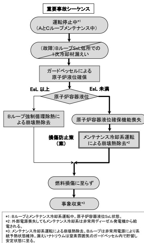
付録 5.1.3 図-3 運転停止中原子炉冷却材の流出の重要事故シーケンス
