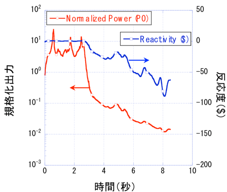
付録 5.2 図-12 「もんじゅ」遷移過程解析ノミナルケースにおける反応度と出力の時間履歴
