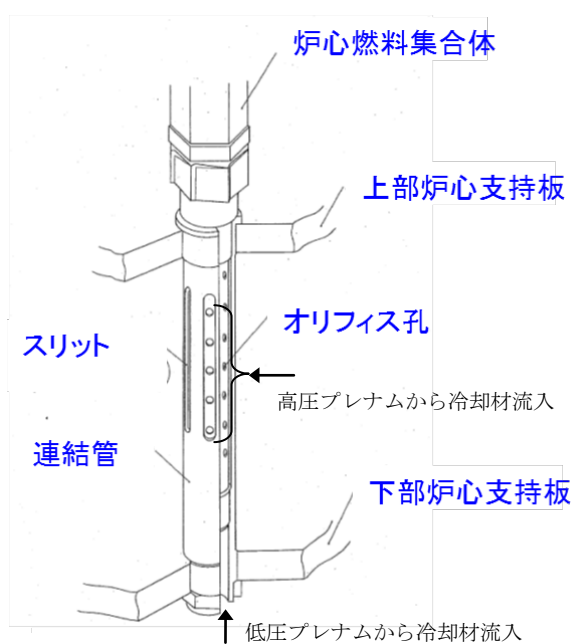
付録 5.1 図-9 「もんじゅ」における集合体入口完全閉塞の防止対策
