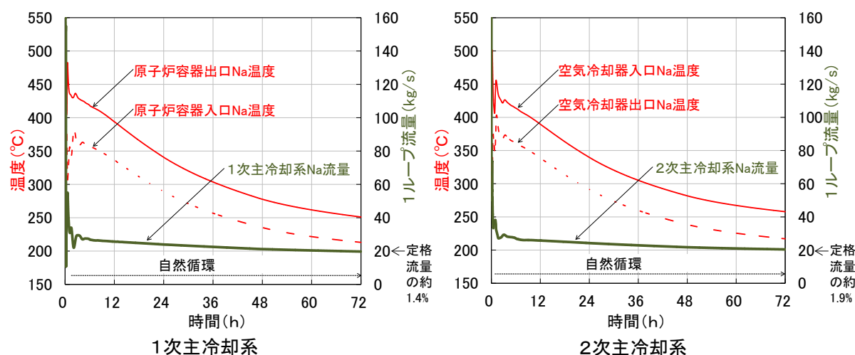
付録 5.1 図-17 全交流動力電源喪失時のプラント過渡応答解析結果例 (2/3)
