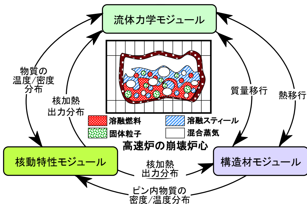
付録 5.2 図-6 遷移過程解析コード SIMMER-III 及び SIMMER-IV の構造
