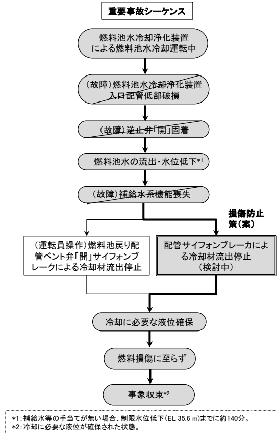
付録 5.1.2 図-7 燃料池の重要事故シーケンス
