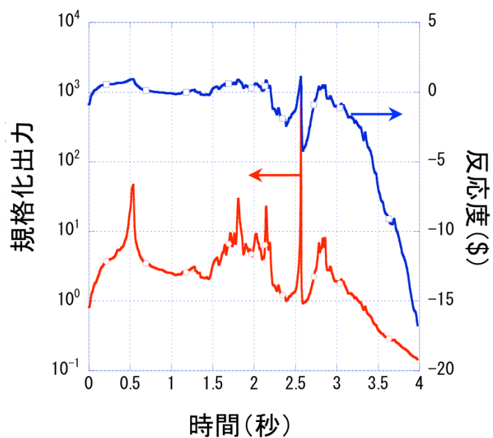
付録 5.2 図-13 「もんじゅ」遷移過程解析保守側ケースにおける反応度と出力の時間履歴
