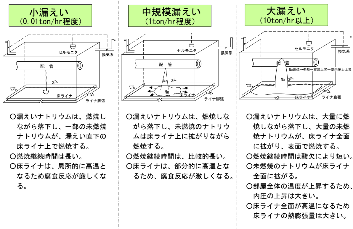
図 3.10.2-2 漏えい規模と漏えいナトリウム燃烧の影響
