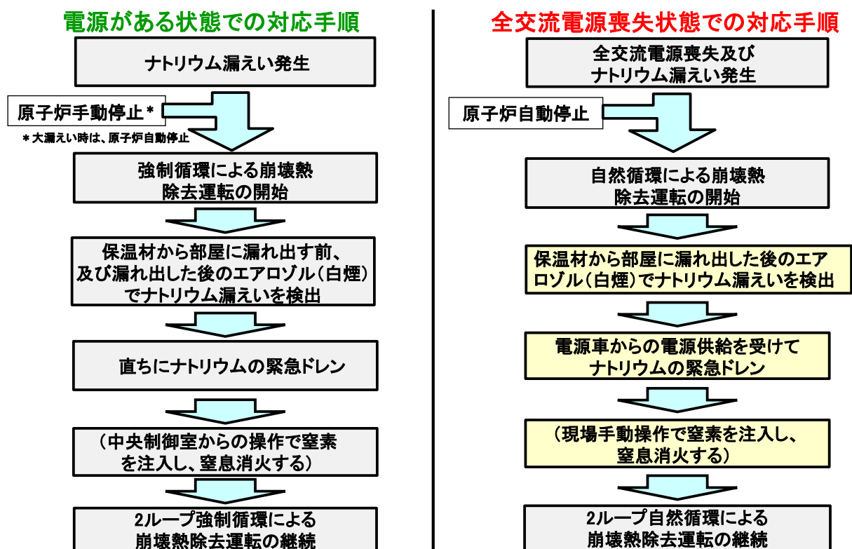
付録 4.2 図-8 電源がある状態での対応手順と、全交流電源喪失状態での対応手順
