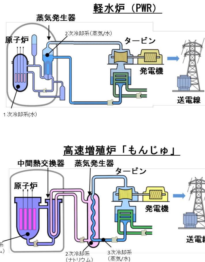
図 2-1 プラントシステム構成の軽水炉と高速炉の比較
