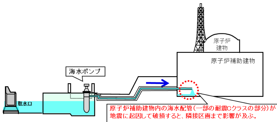
図 3.6-4 建物内海水配管の耐震補強箇所
