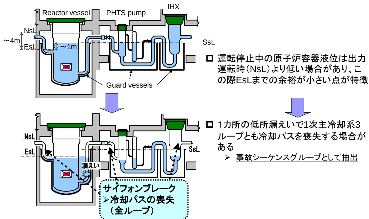
付録 5.1.3 図-1 運転停止中(メンテナンス中)の原子炉容器ナトリウム液位
