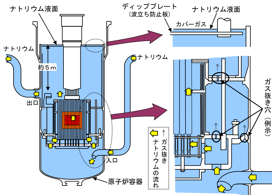
付録 5.1 図-10 「もんじゅ」における気泡対策
