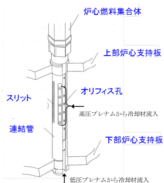
図 4.2.1-8 「もんじゅ」における集合体入口完全閉塞の防止対策
