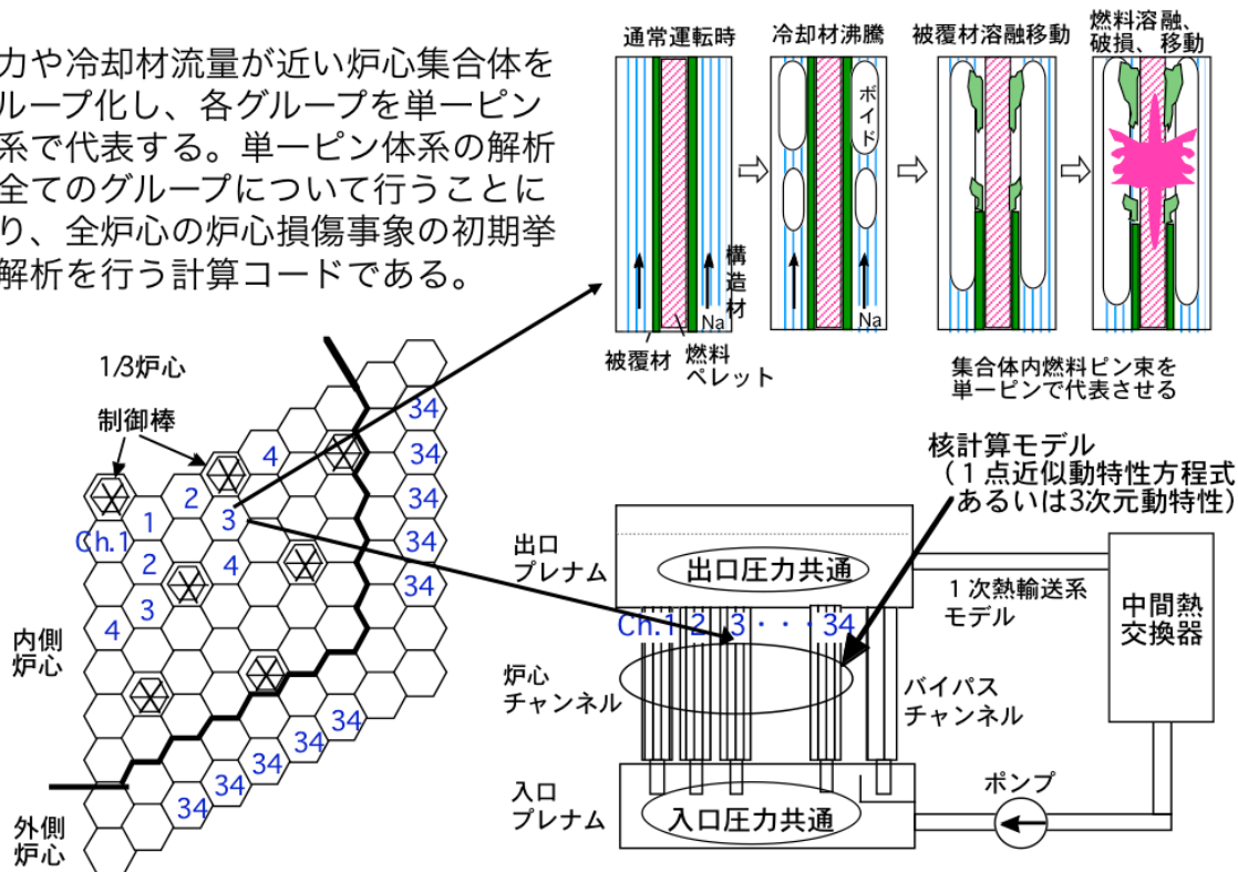
付録 5.2 図-2 SAS4A コードの概要
