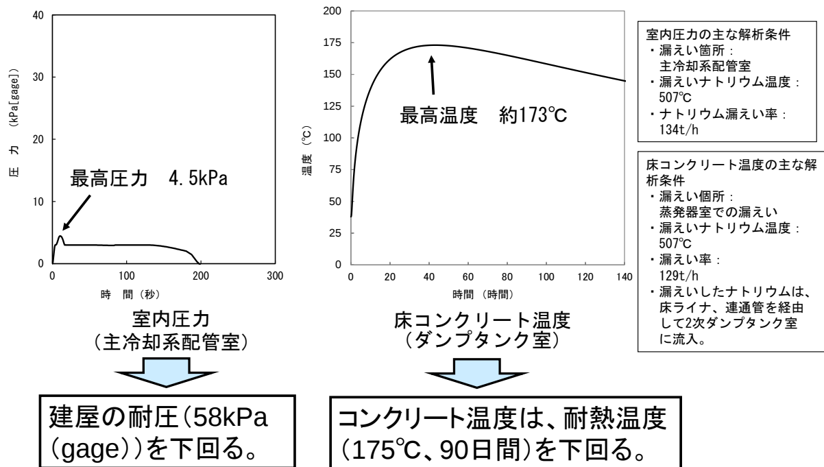
付録 4.2 図-11 全交流電源喪失状態での評価結果（発生圧力・コンクリート温度）
