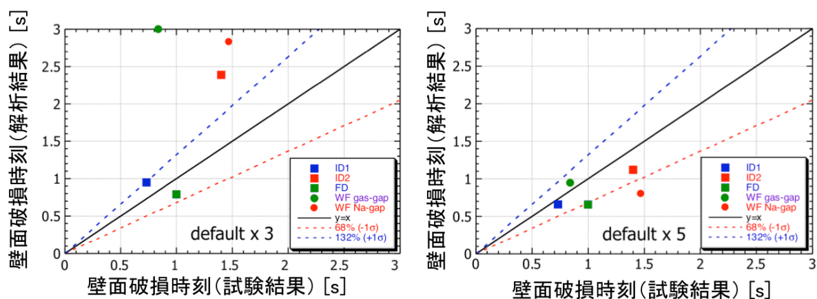
付録 5.2 図-9 EAGLE 炉内試験の壁破損時刻の SIMMER-III による解析結果
