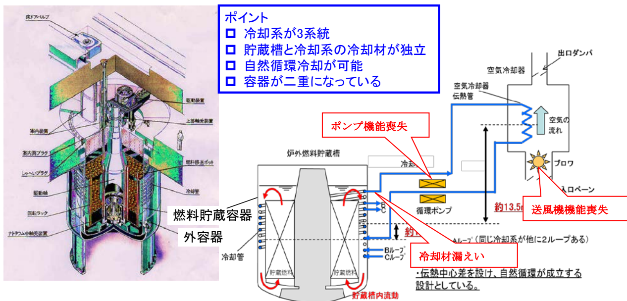
付録 5.1.2 図-1 炉外燃料貯蔵槽(EVST)の概要
