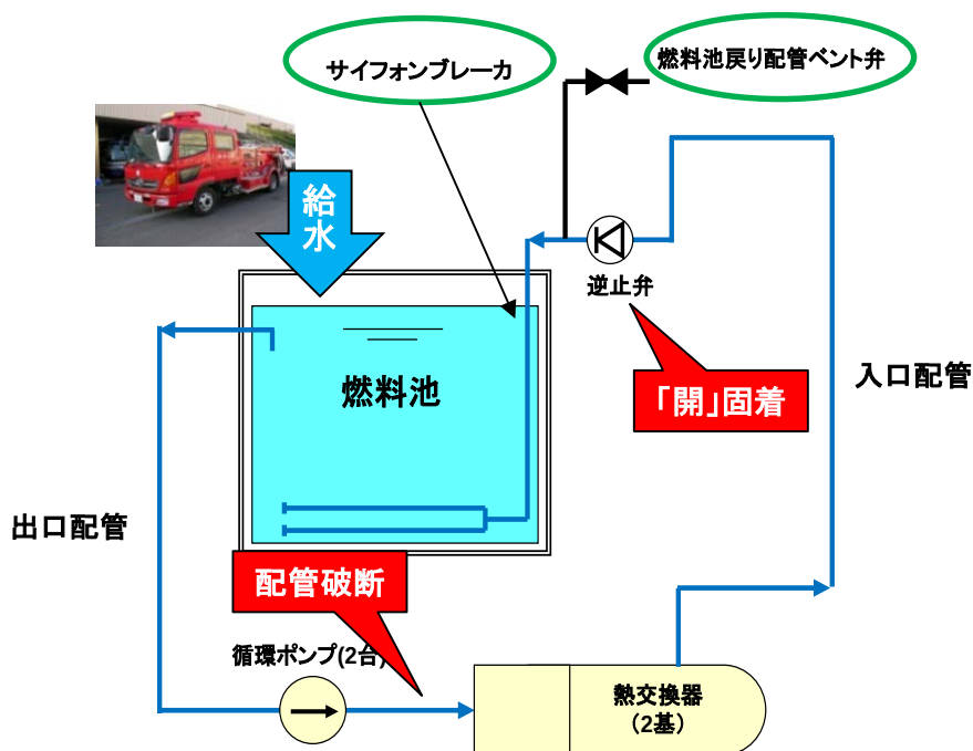
付録 5.1.2 図-4 燃料池の重要事故シーケンスと損傷防止策
