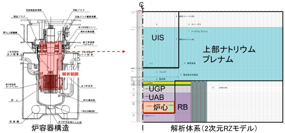
付録 5.2 図-14 「もんじゅ」炉容器応答過程における炉心膨張挙動解析体系
