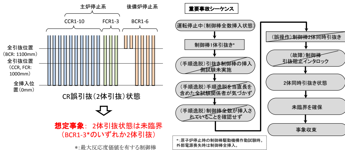
付録 5.1.3 図-2 運転停止中反応度誤投入の重要事故シーケンス
