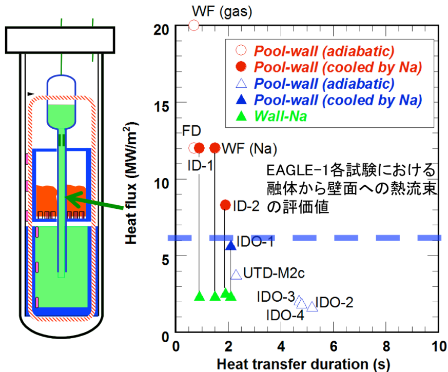
付録 5.2 図-8 EAGLE 試験の炉内試験例(ID-1 試験)
