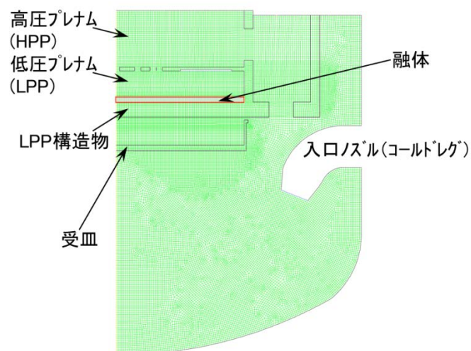
付録 5.2 図-18 FLUENT コードによる「もんじゅ」下部プレナム流動状況解析体系
