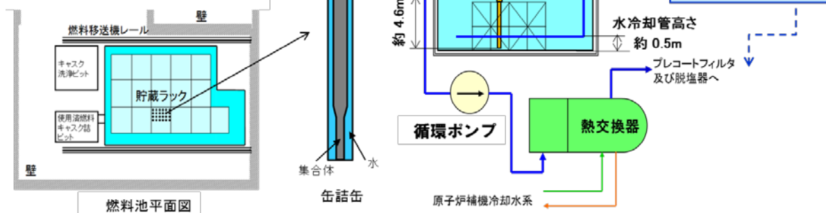
図 4.2.2-3 燃料池の概要
