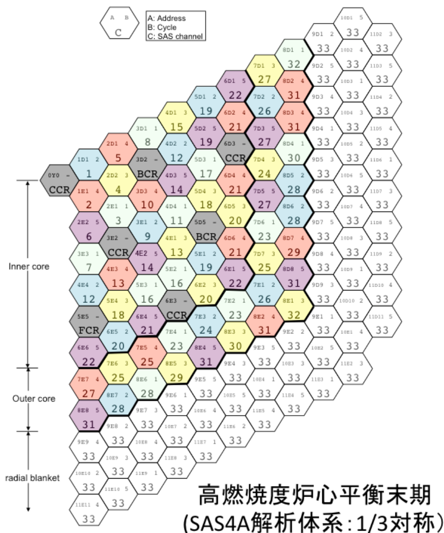
付録 5.2 図-3 「もんじゅ」起因過程解析のチャンネル割り当て
