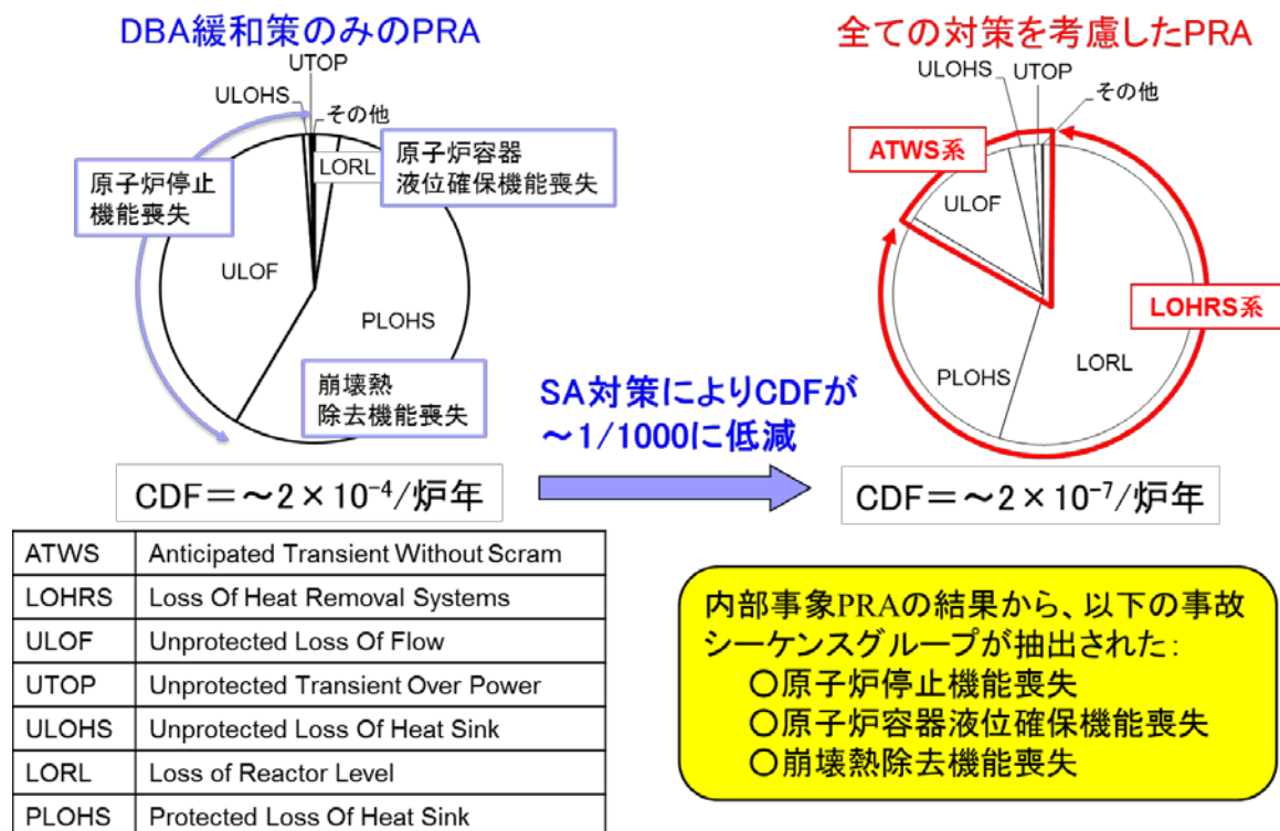
付録 5.1 図-2 内部事象から選定される事故シーケンスグループ(レベル1PRAの結果)
