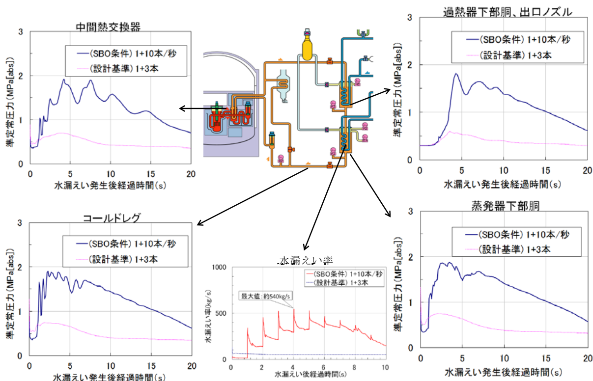
付録 4.1 図-12 設計基準の水漏えい規模を超える想定での水漏えい率と発生圧力
