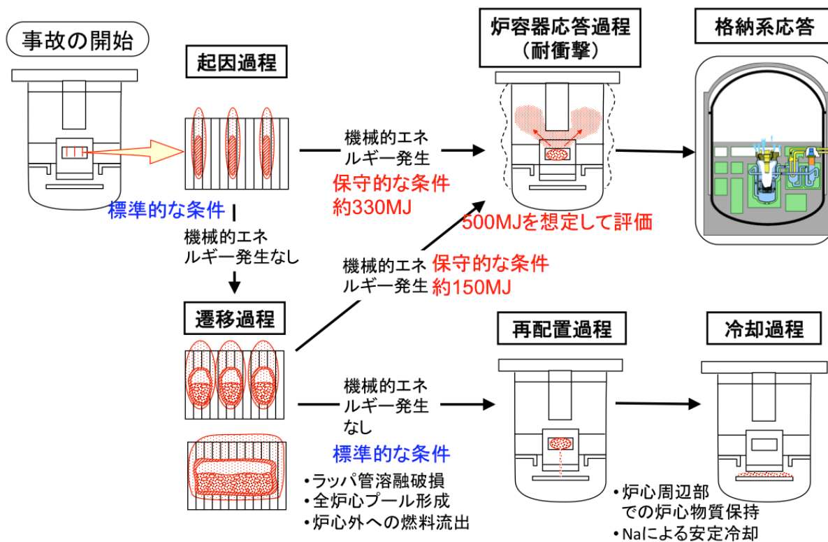
図 2-3 ULOF 事象の事象推移の概要
