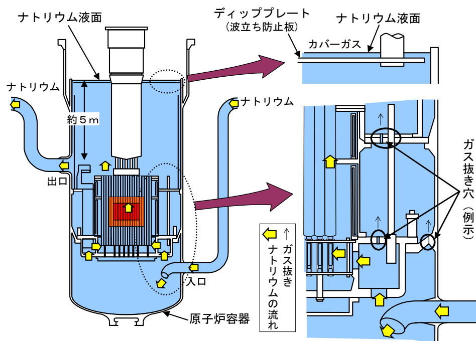
図 4.2.1-9 「もんじゅ」における気泡対策
