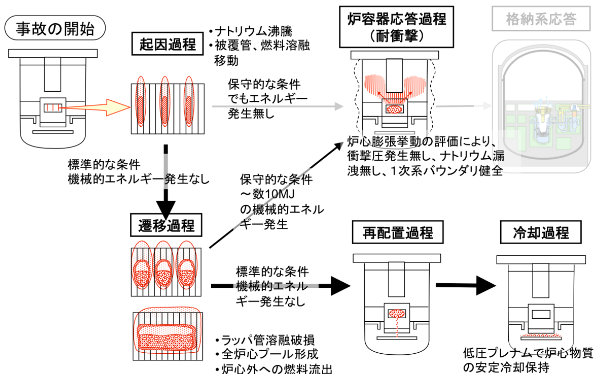
付録 5.2 図-1 ULOF 事象推移評価の概要
