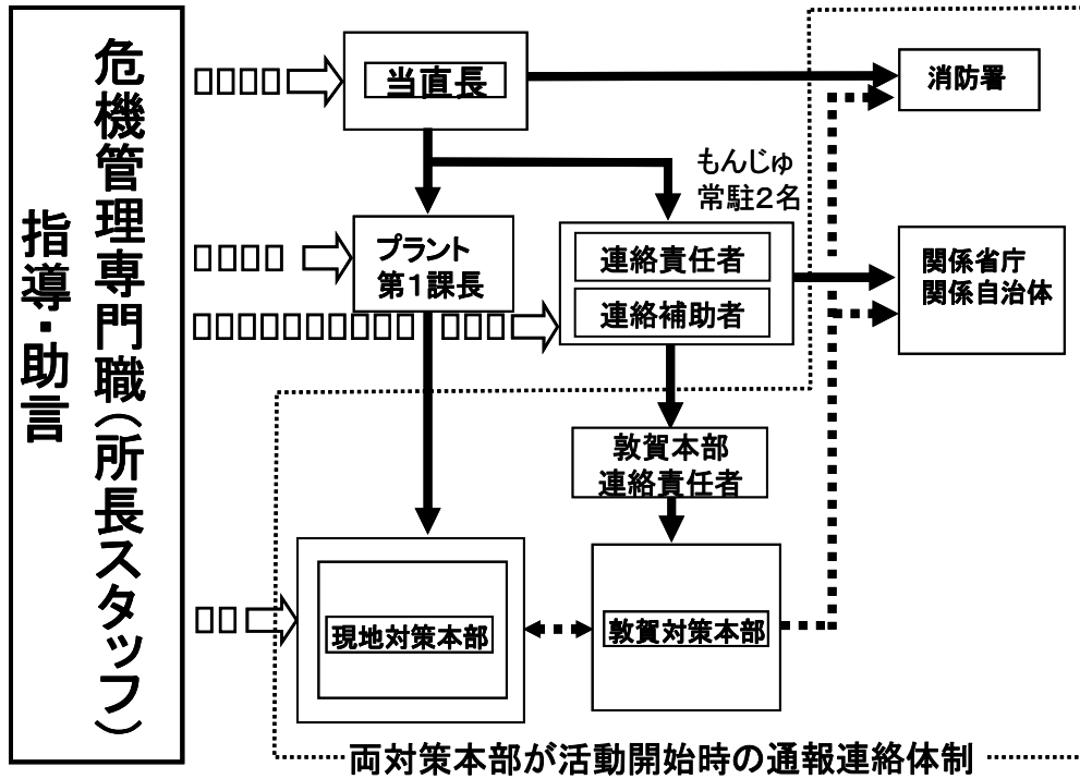
体制図
