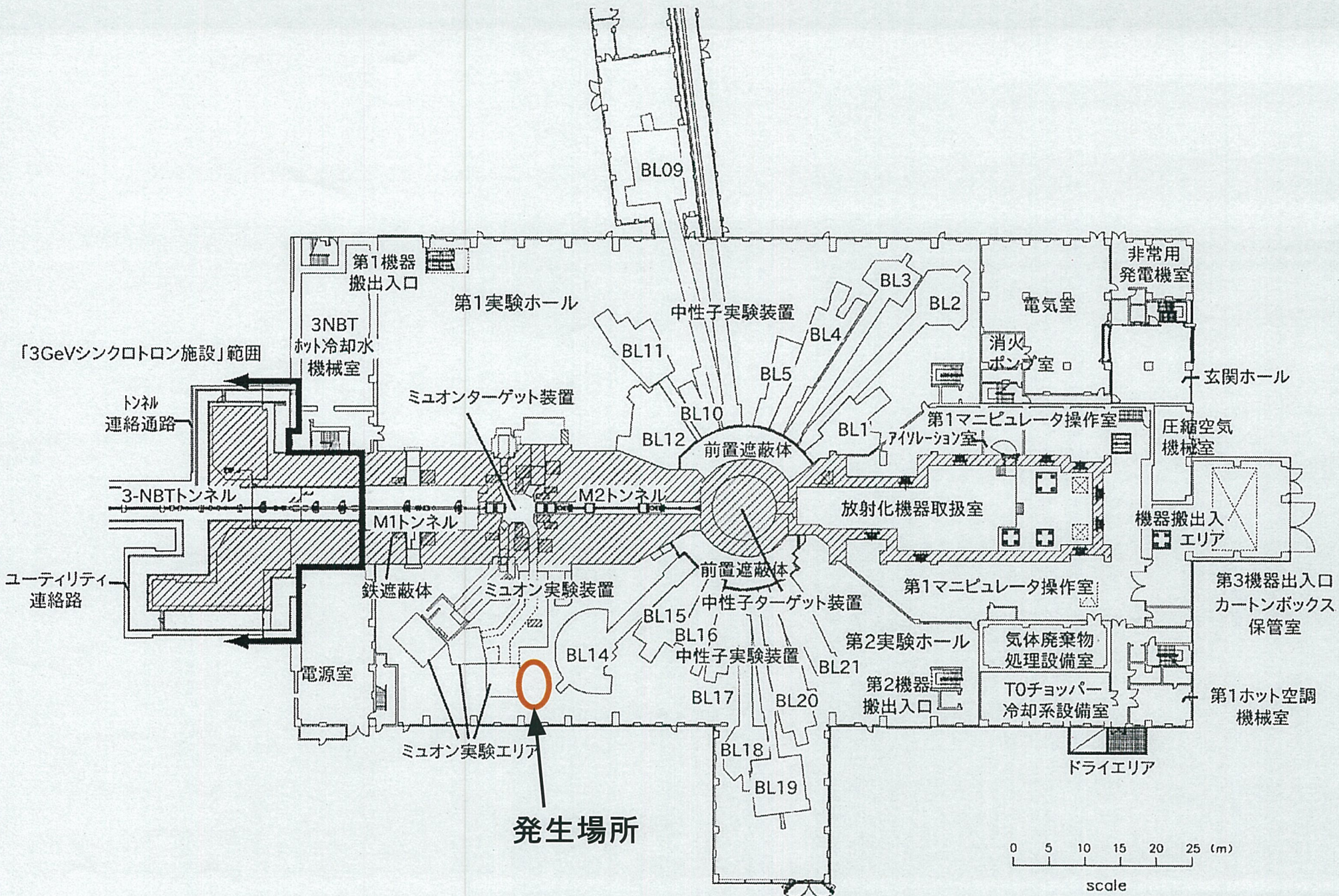
物質・生命科学実験施設 平面図 (1階)
