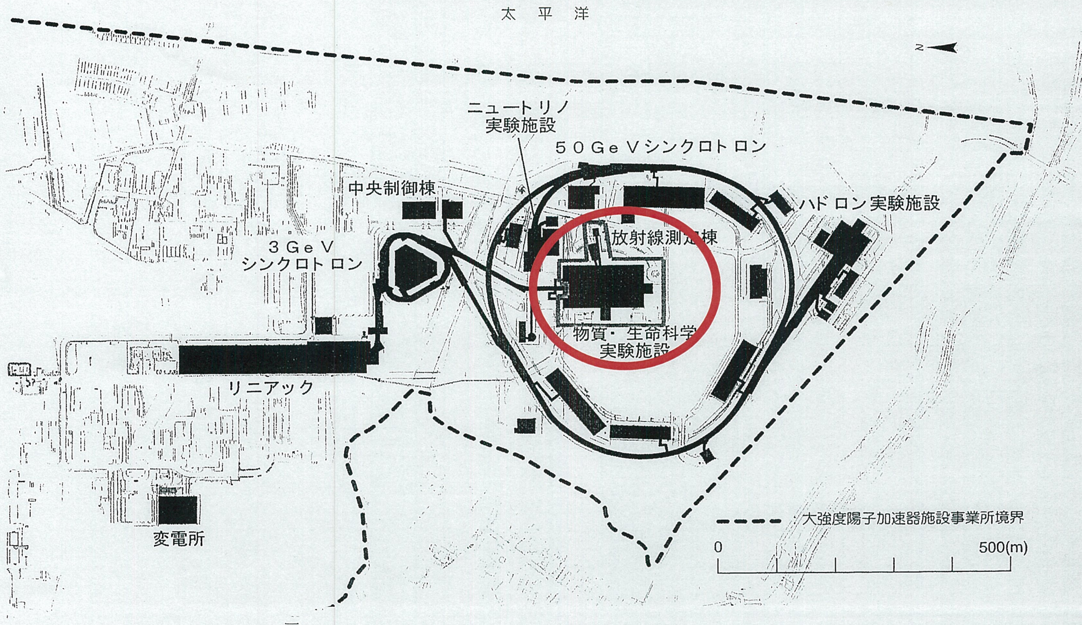
図1 大強度陽子加速器 (J-PARC) 物質・生命科学実験施設
