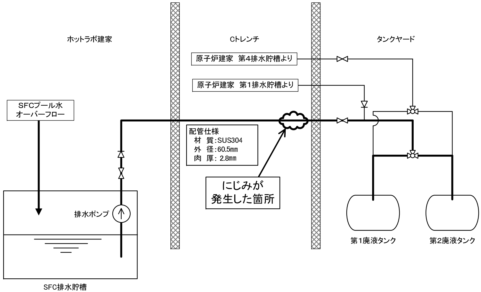
図3 SFC 排水貯槽廃液移送系統図
