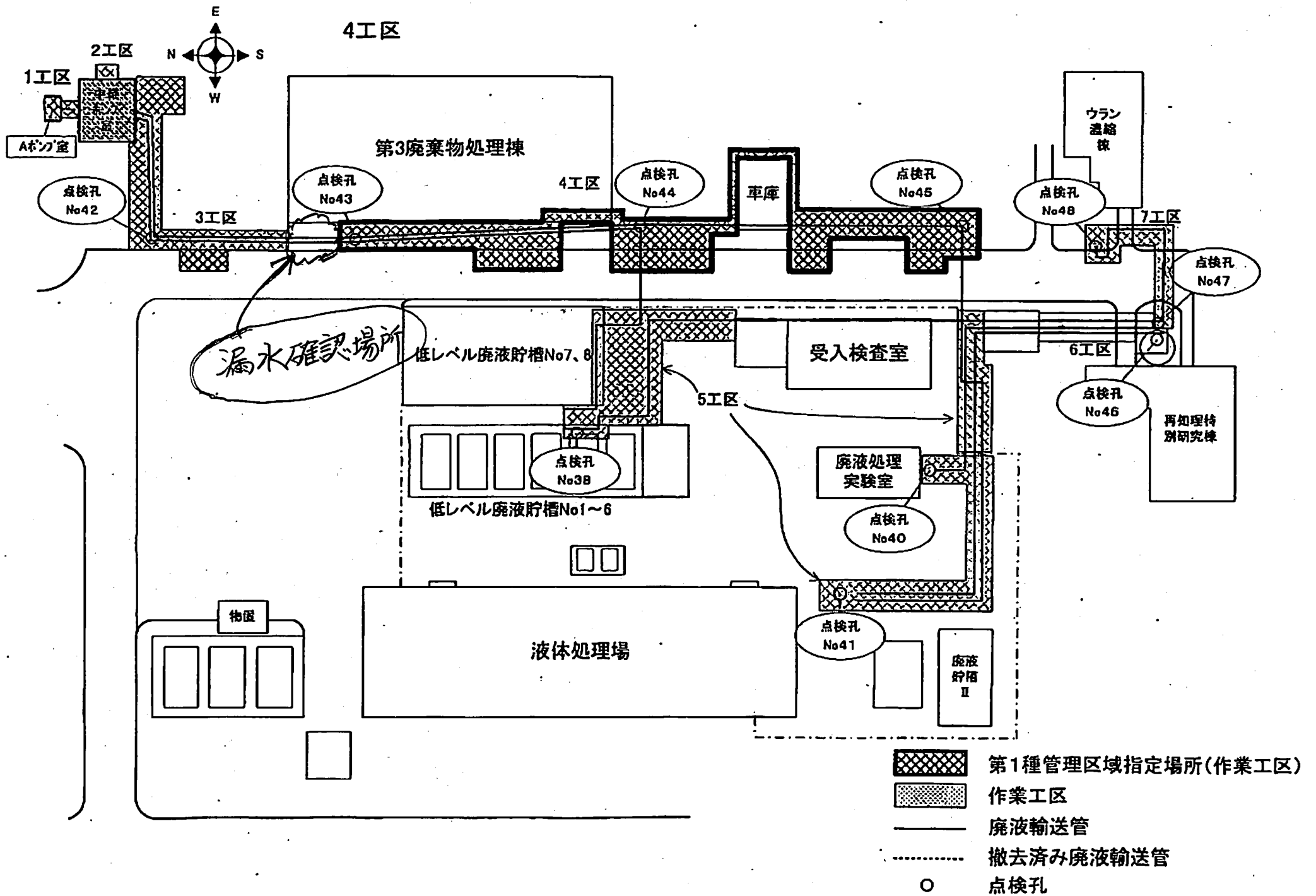
添付資料 廃液輸送管撤去に係わる第1種管理区域指定場所 配置図
