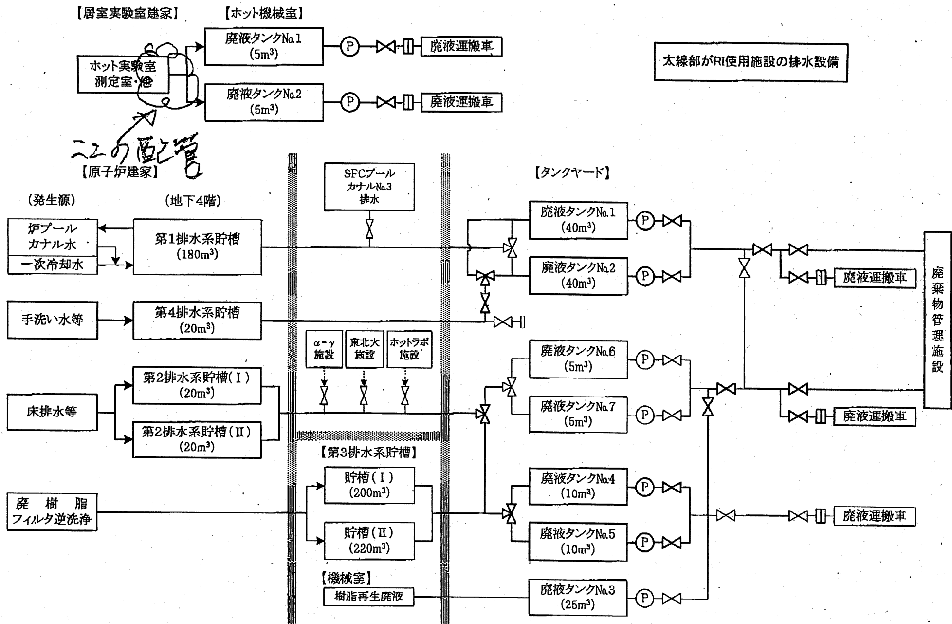
居室実験室及び原子炉建家の排水設備の概要図
