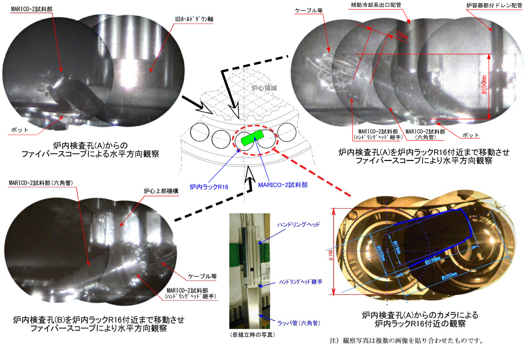
別添図3 炉内ラックR16上部のMARICO-2試料部観察写真
