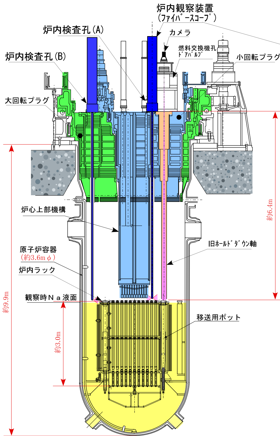
別添図2 原子炉容器内の観察概要図
