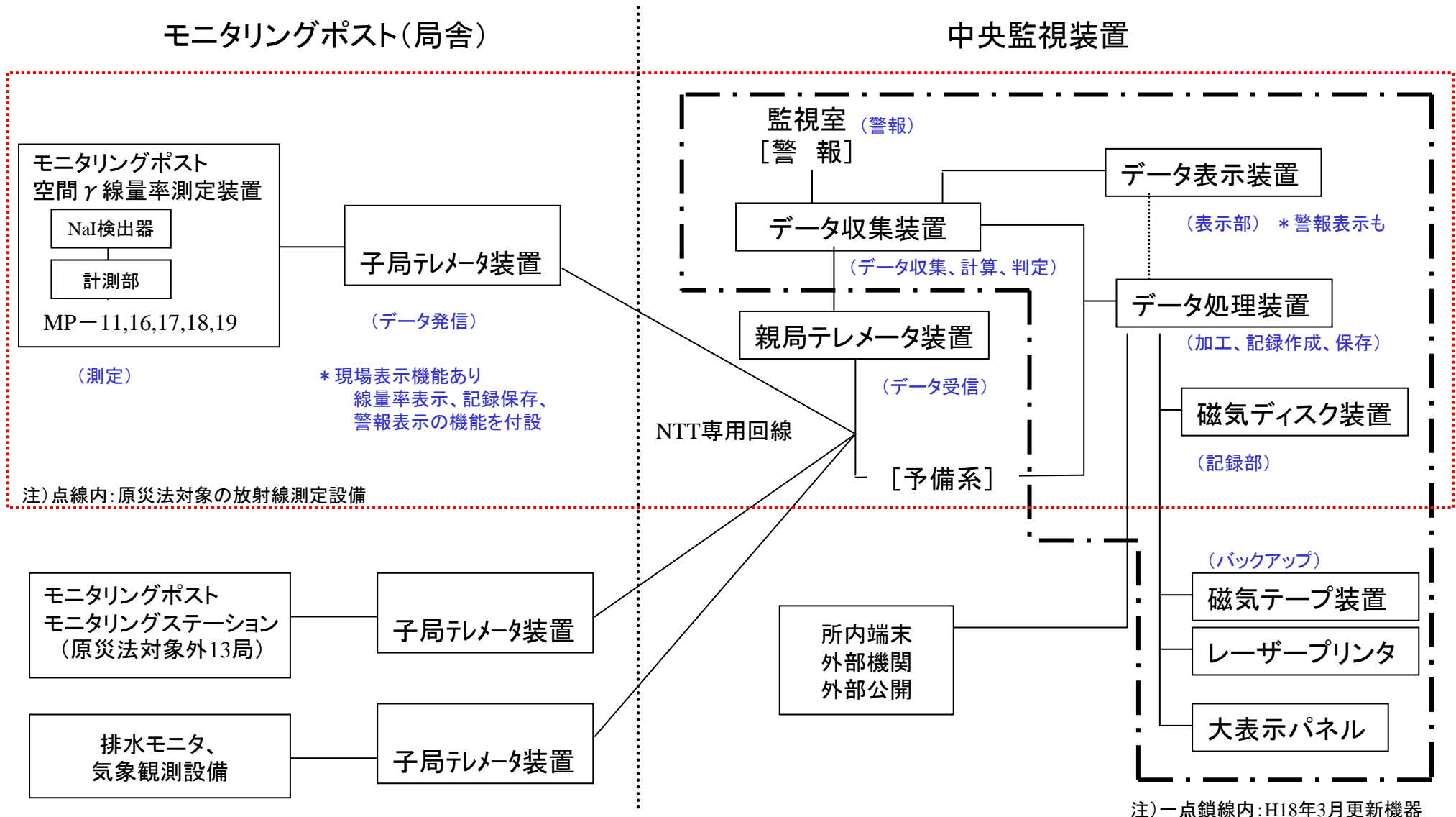
図1 原子力科学研究所の放射線測定設備の構成
