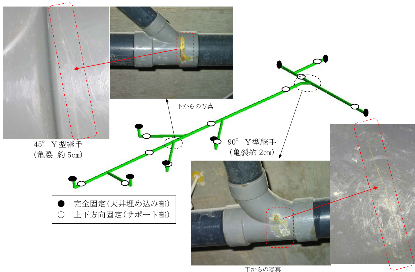
図-3 資材一時置場分析廃水配管継手の亀裂調査結果
