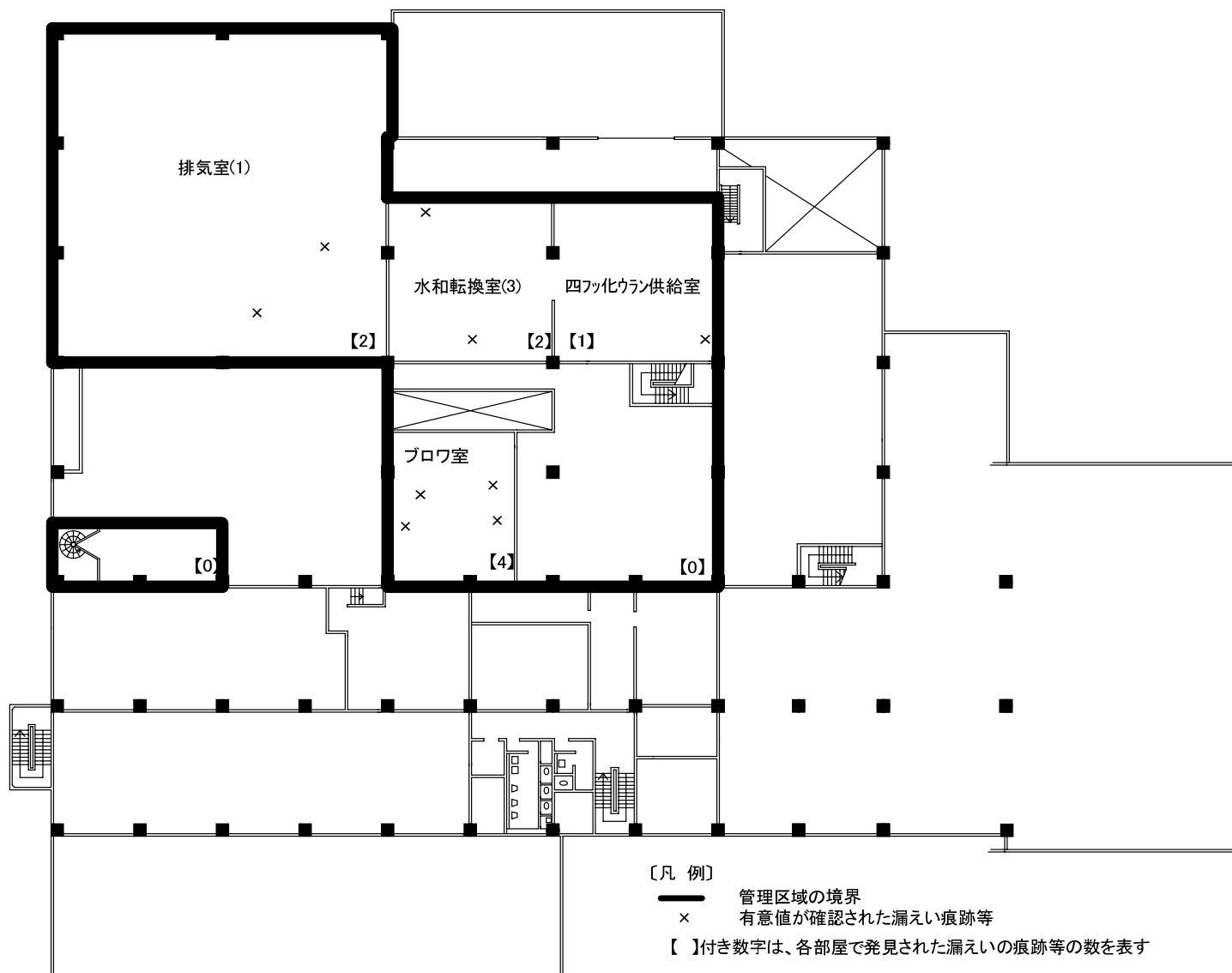
図-1.3 部屋別の漏えい痕跡箇所（3階）
