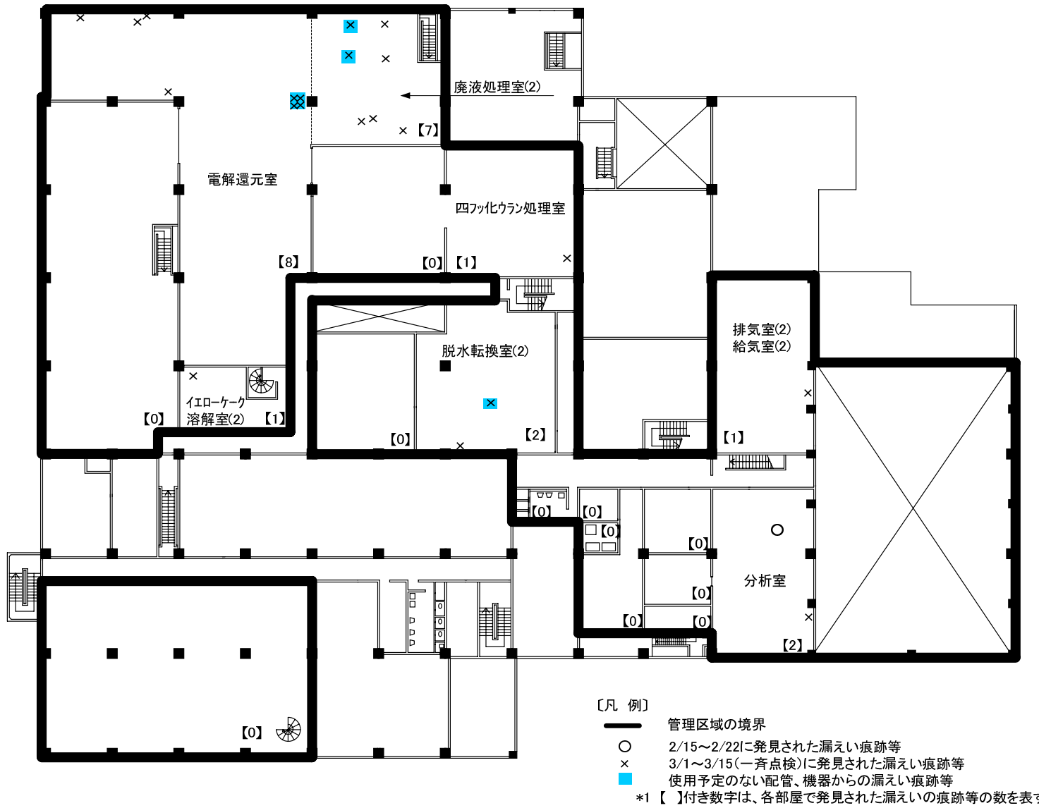
図-1.2 部屋別の漏えい痕跡箇所 (2階)
