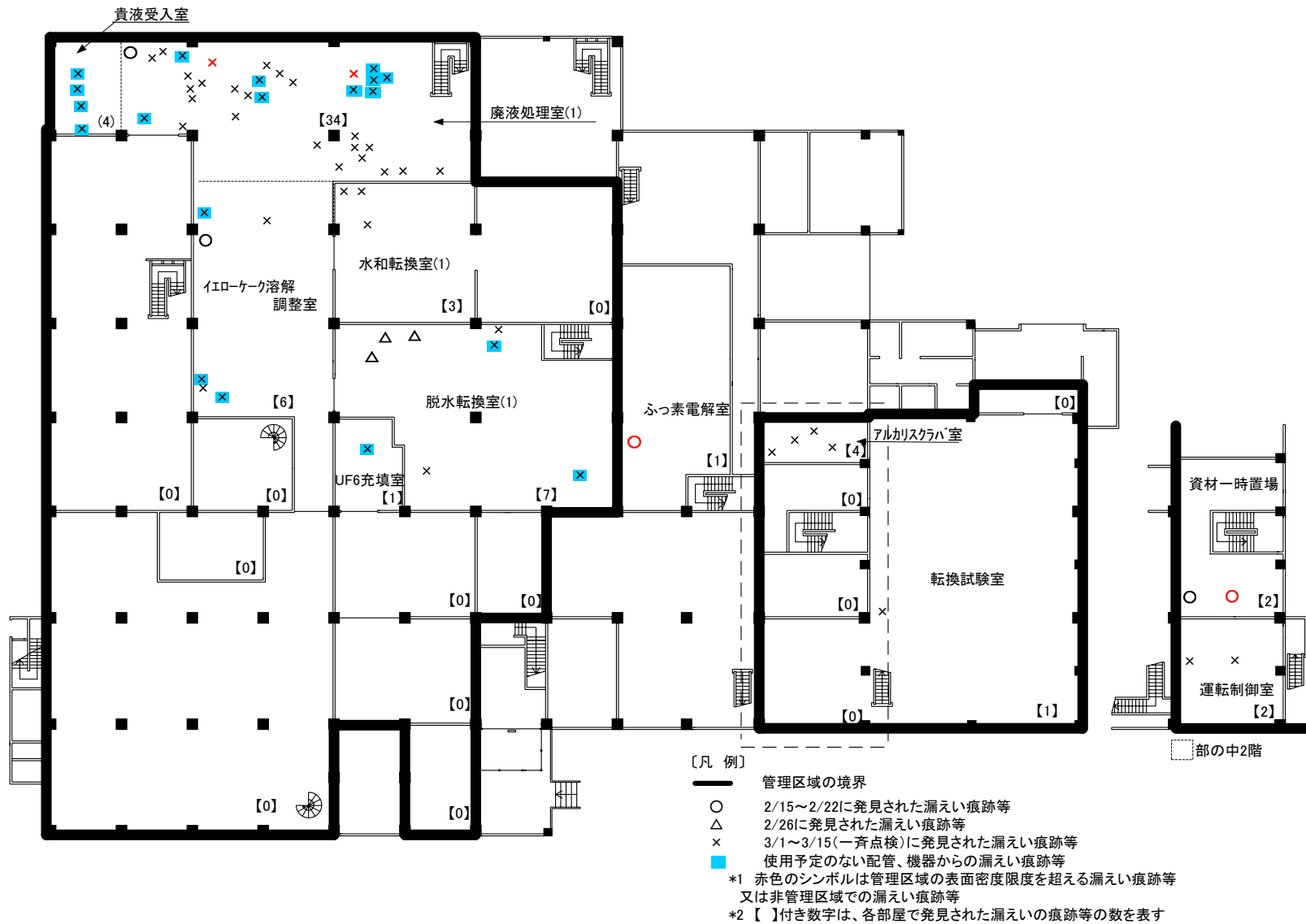
図-1.1 部屋別の漏えい痕跡箇所 (1階・中2階)
