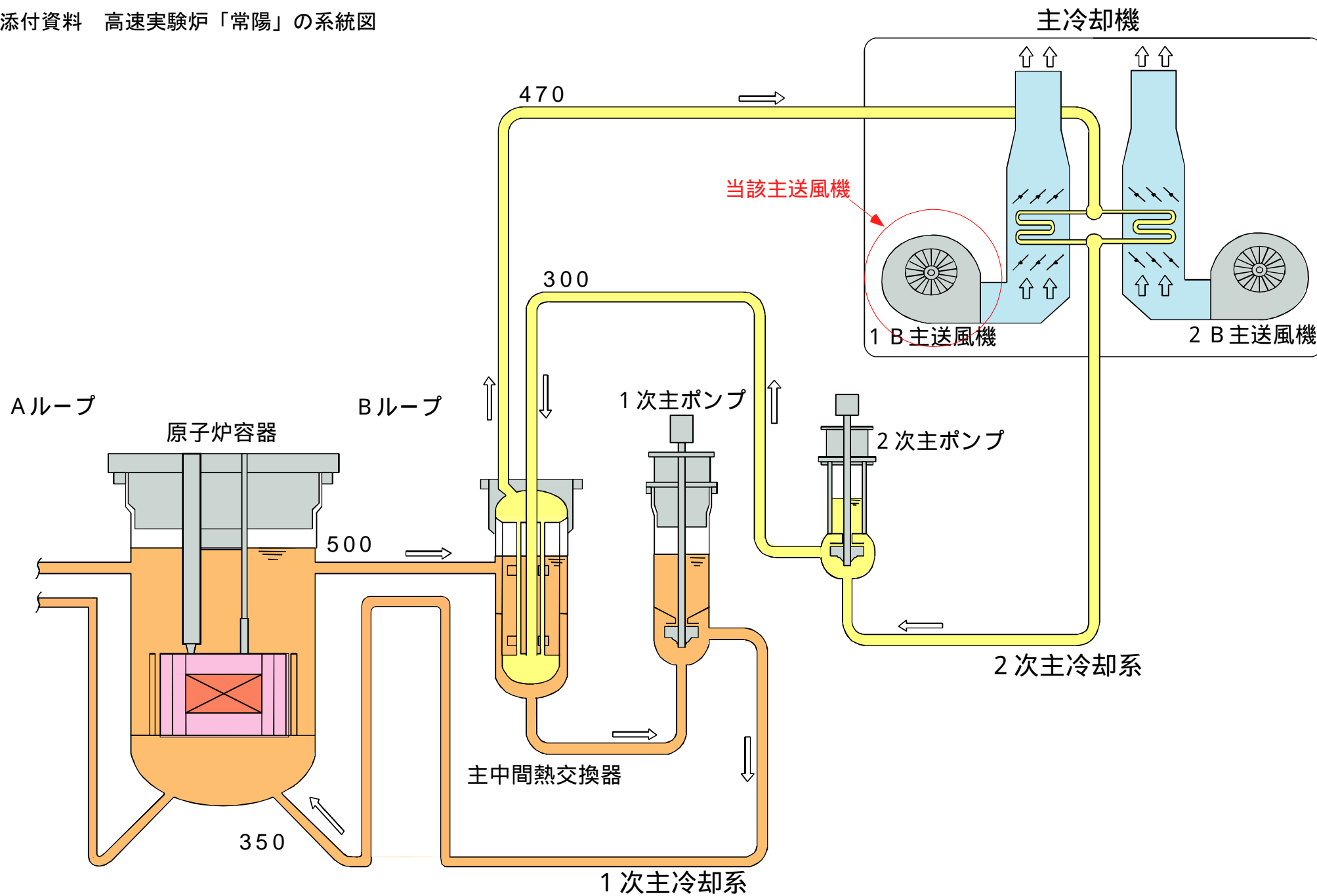
高速実験炉「常陽」系統図
