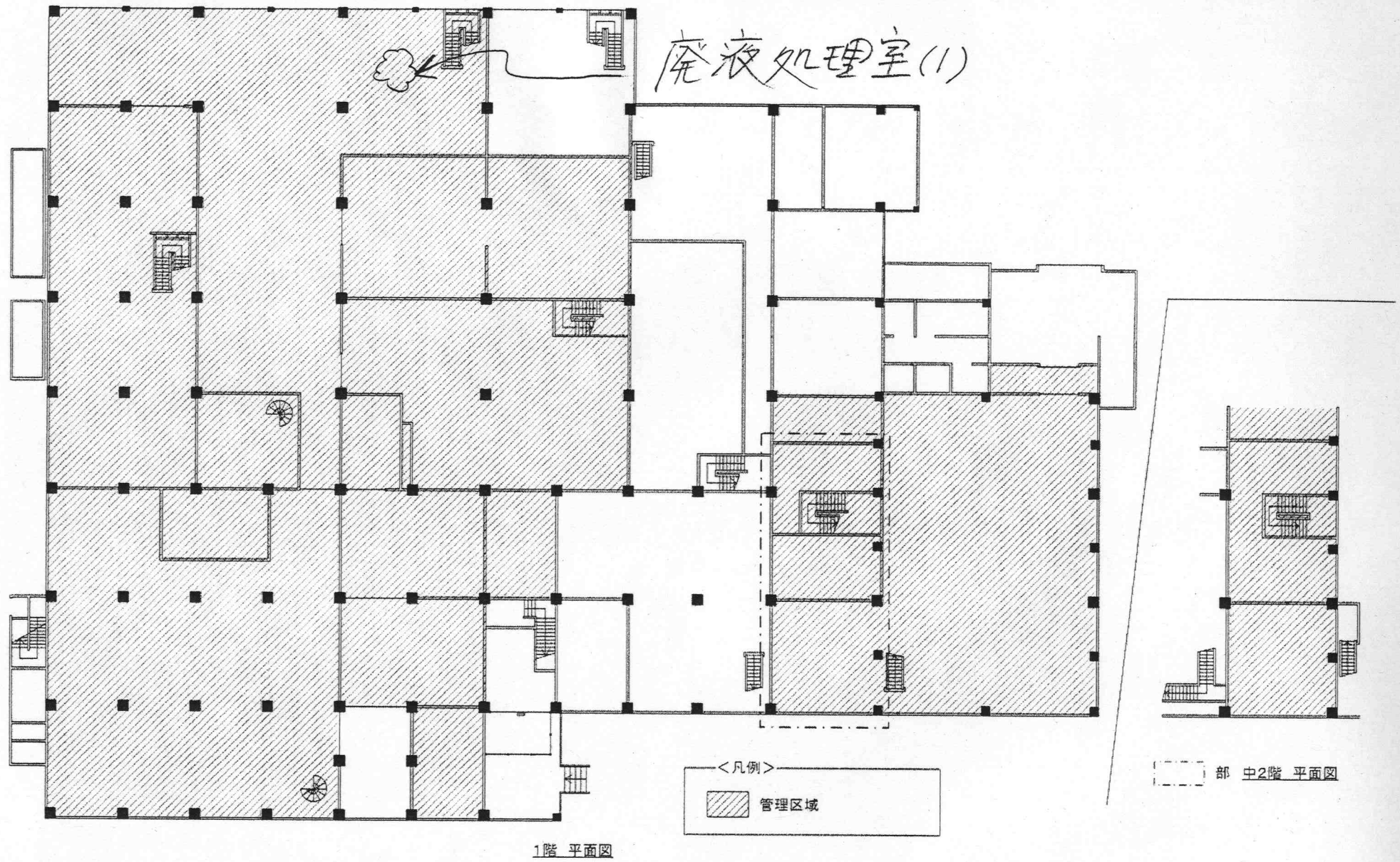
図-2 製鍊轉換施設一階及び中二階平面図
