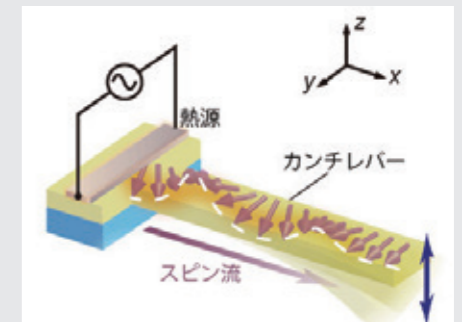
本研究に用いた装置の概略図
