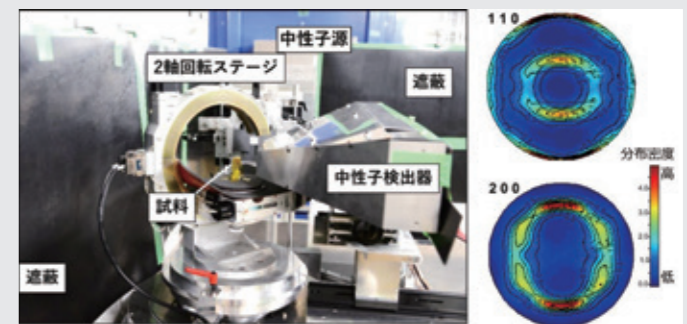
小型中性子源システムを用いた鉄鋼材料の集合組織測定実験の様子と結果
