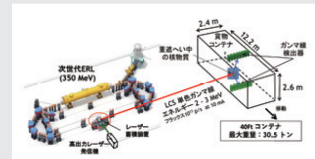
(例) 40フィート輸送コンテナの非破壊検査へのNRF技術の適用
