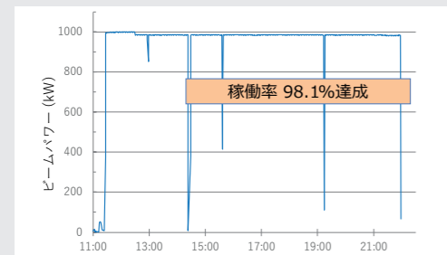
1MW相当のビームパワーによる利用運転時の履歴
