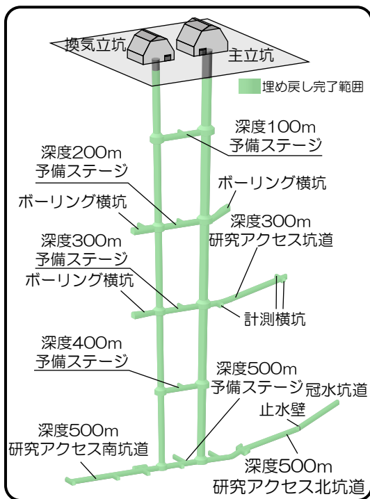
【坑道埋め戻し状況】 (令和3年10月19日現在)
