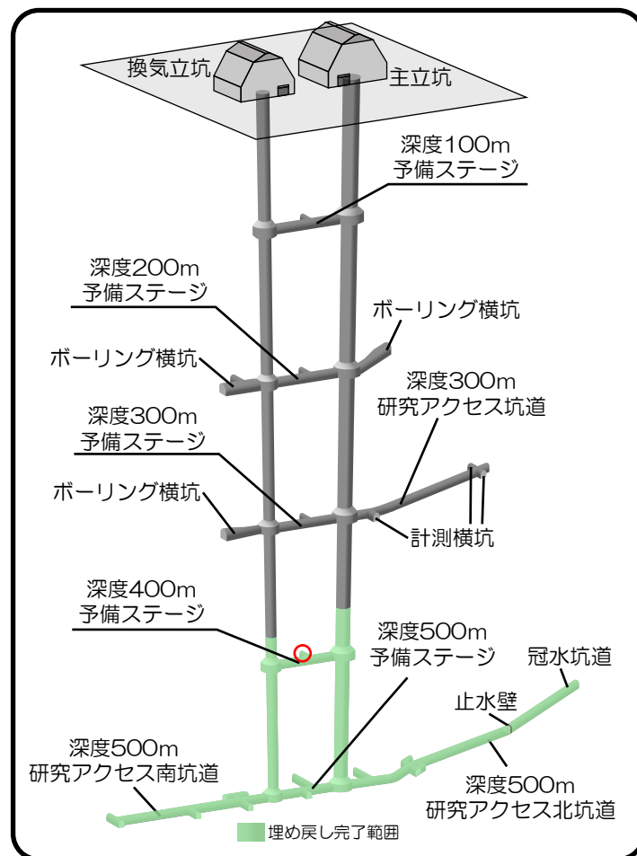
坑道埋め戻し状況（2020.10.16現在）
