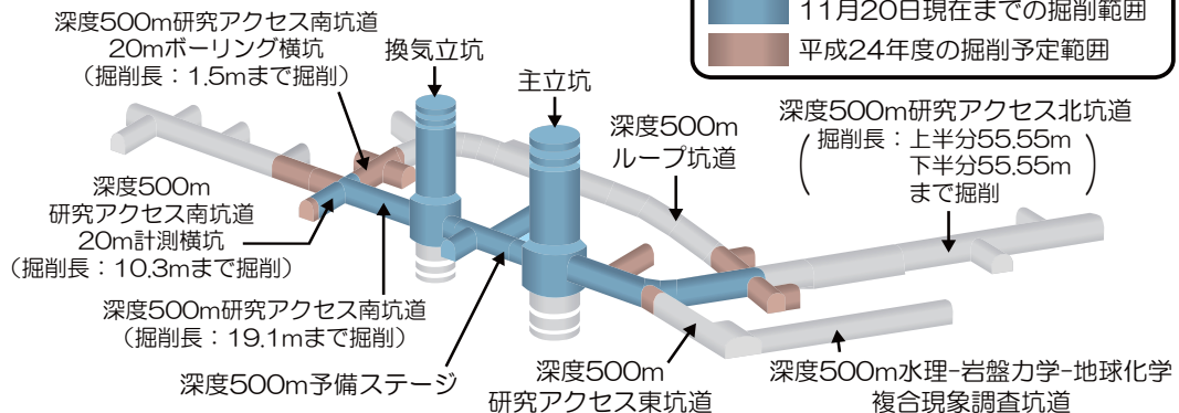
【瑞浪超深地層研究所 深度500mステージのイメージ図】
