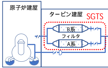
SGTSの概略図
