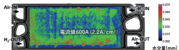
トヨタ自動車の新型MIRAIに搭載される燃料電池セル(写真上)と稼働中の水の生成・排出挙動(写真下)
