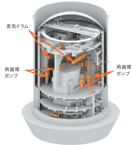
大型機器解体撤去対象範囲
