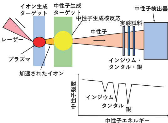
レーザー中性子源の原理
