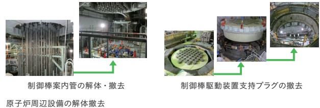
原子炉周辺設備の解体撤去
