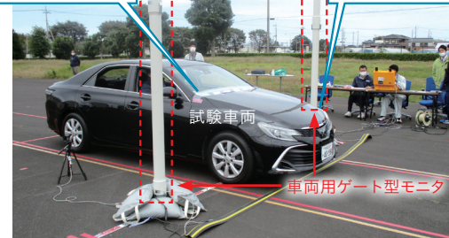
可搬型ゲート型モニタを使用した車両測定実験の様子
