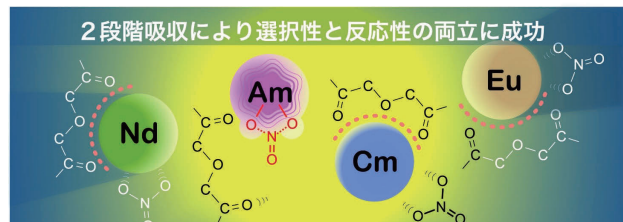
レーザーアシスト元素分離の概念
